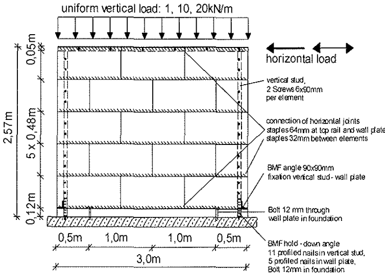
Fig. 7 PFTE Test Wall Specimen
