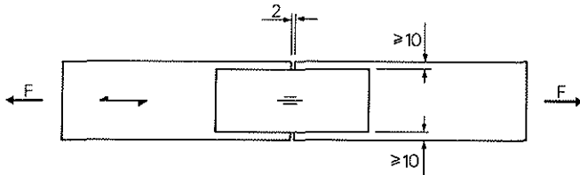
Fig. 3. - Éprouvette pour l'essai de la résistance à la traction de la plaque. \alpha=0 et 90^\circ ; \beta=0^\circ .
