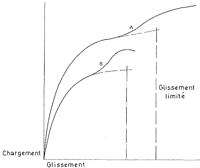
Fig. 9. – Courbes chargement-cisaillement pour l'essai de cisaillement ; les courbes sont extrapolées de la limite apparente d'élasticité pour donner des valeurs supposées de la charge maximale A où la charge maximale n'est pas notée avant d'atteindre le glissement limite approprié et B où la charge maximale d'essai est notée à une valeur de glissement inférieure à la valeur limite.
