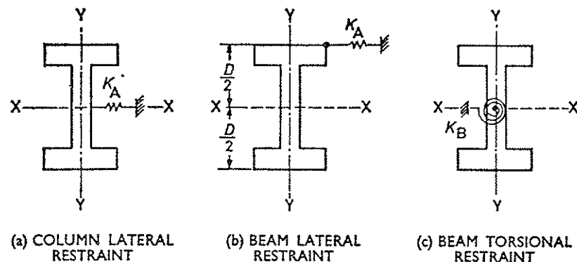
Fig. D1. INTERMEDIATE RESTRAINTS
