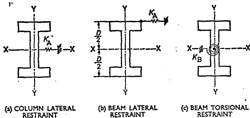
Fig. D1. INTERMEDIATE RESTRAINTS
