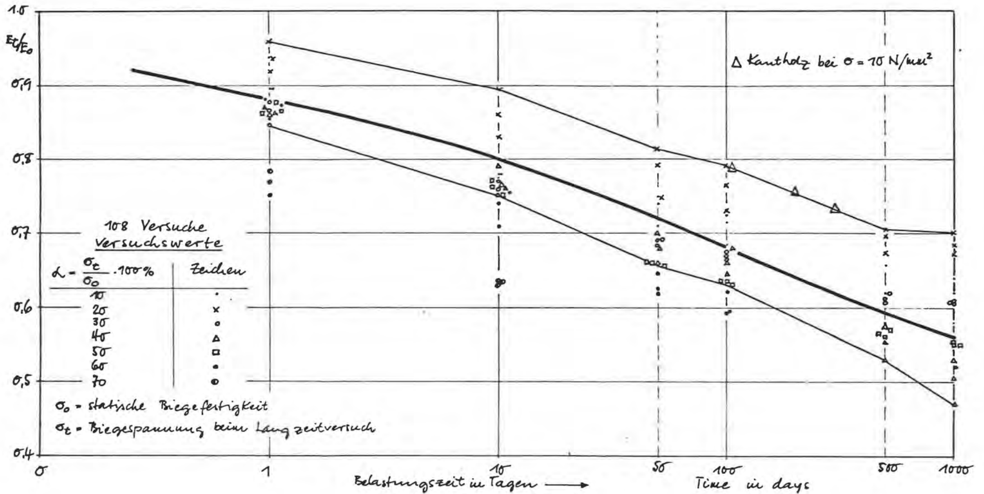
Biegeversuche E_t/E_0 - Zeit - Abhängigkeit bei liegenden Jahrringen
