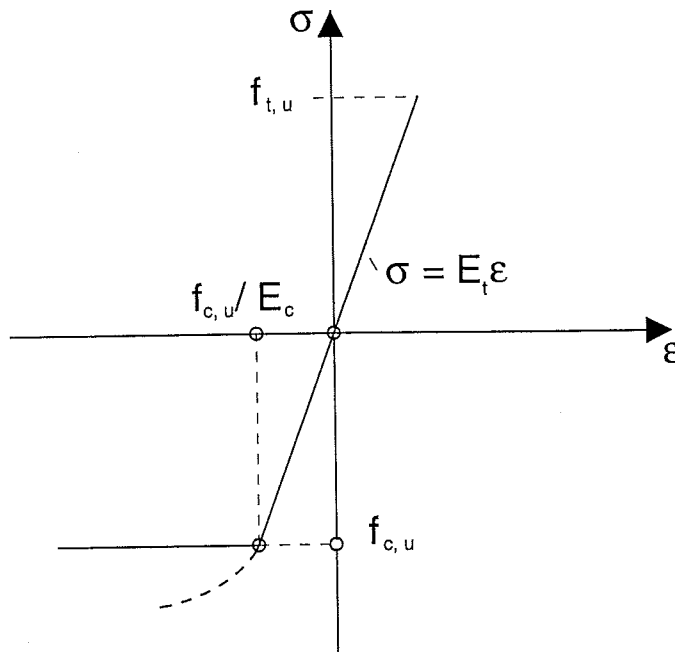
Bild 5.2.5: Angenommenes Spannungs-Dehnungsverhalten
