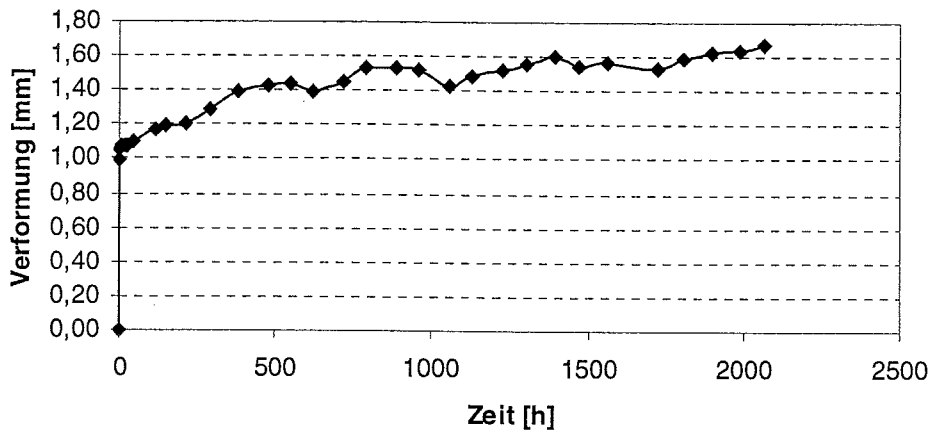
Bild 6.7: Mittelwert der Verformungen im querkraftfreien Bereich des Trägers LT_2
