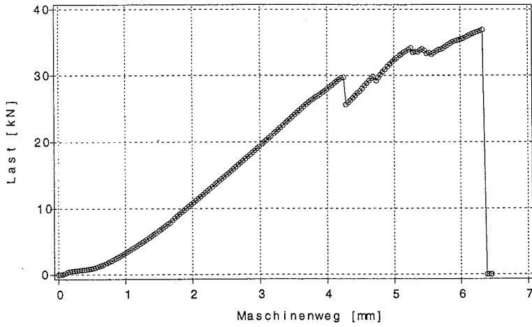
Bild B.79: Last-Verschiebungsverhalten des Prüfkörpers z3a4_4
