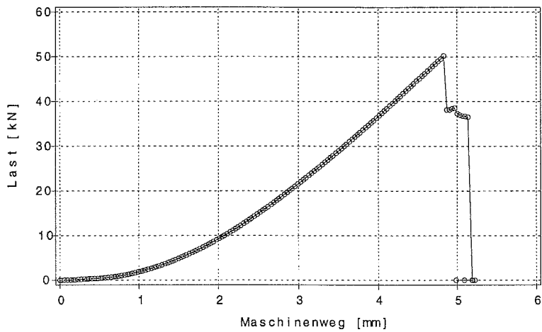
Bild B.59: Last-Verschiebungsverhalten des Prüfkörpers z2b4_4
