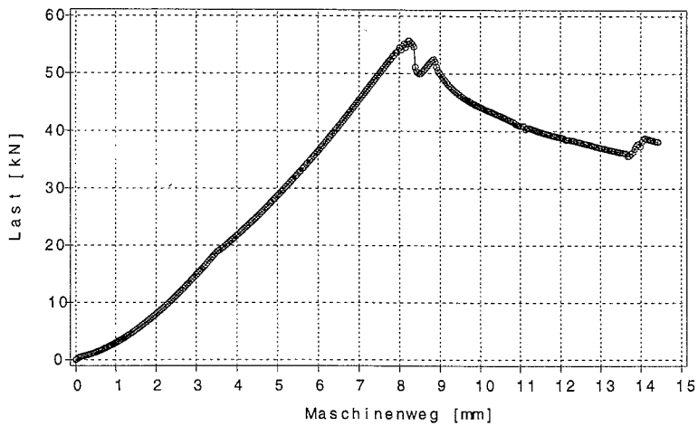
Bild B.58: Last-Verschiebungsverhalten des Prüfkörpers z2b4_3e
