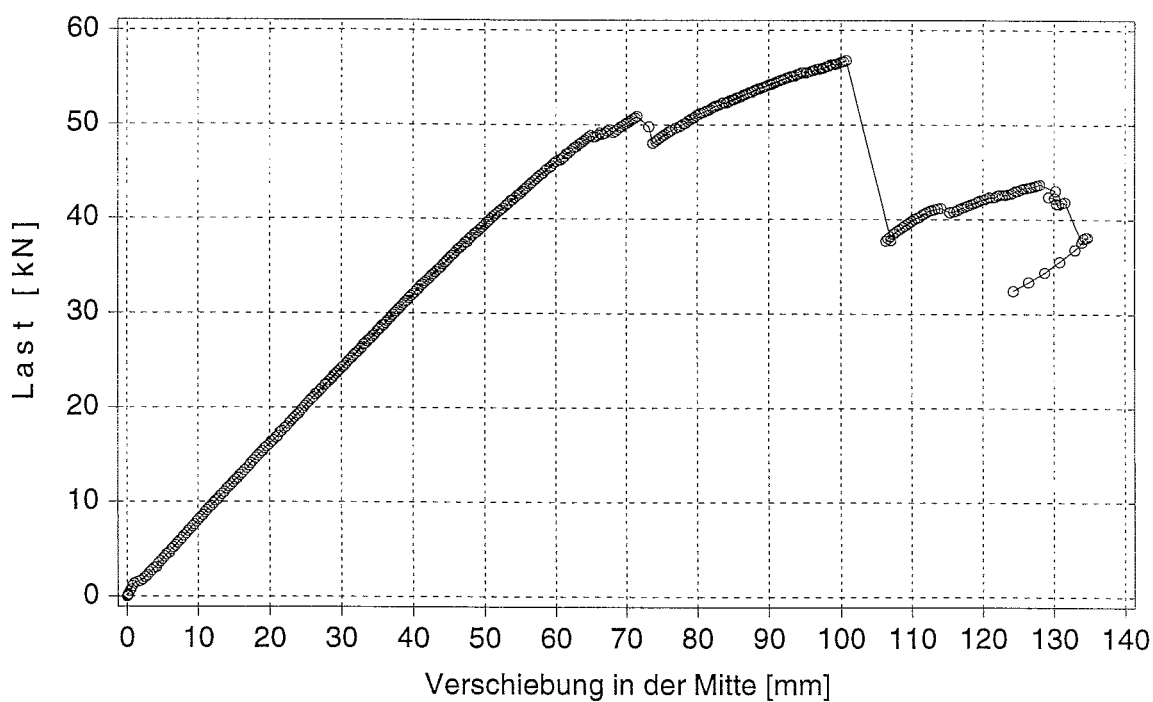
Bild C.4: Last-Verschiebungsdiagramm des Prüfkörpers KT_1_4 (T4)
