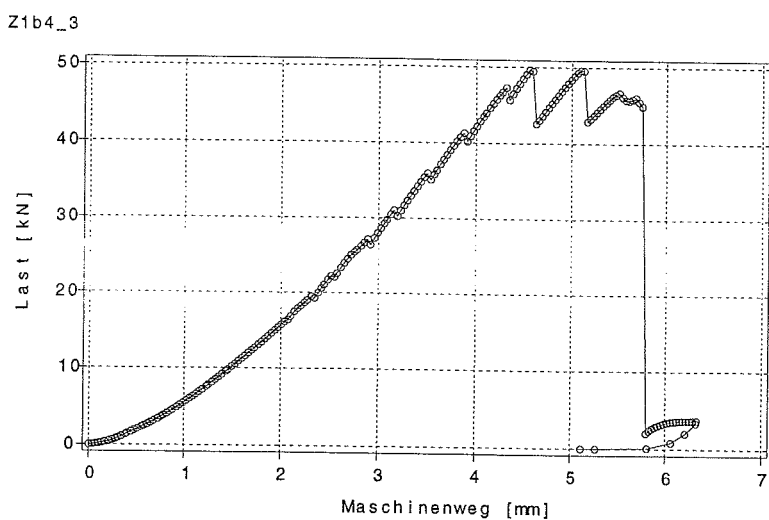
Bild B.18: Last-Verschiebungsverhalten des Prüfkörpers z1b4_3
