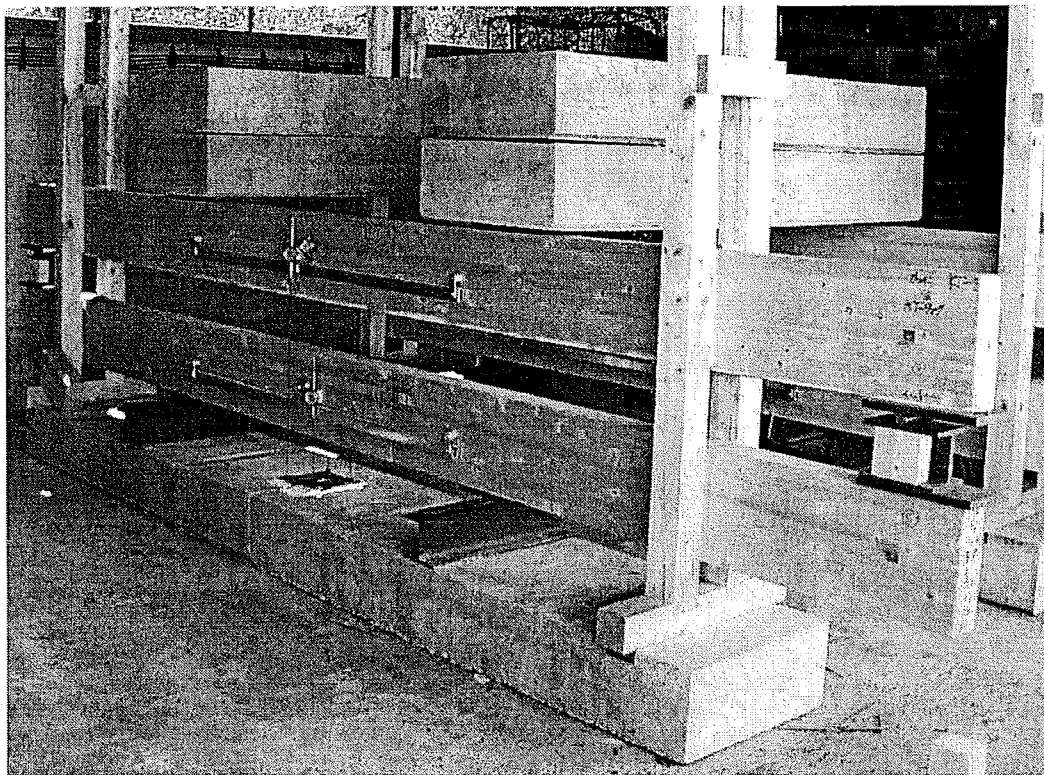
Bild 6.4: Seitenansicht des Versuchsaufbaus
