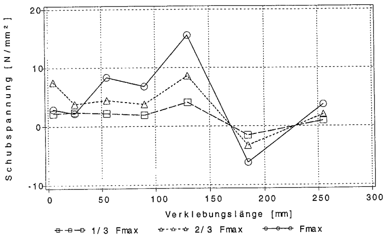
Bild B.110: Schubspannungsverläufe des Prüfkörpers z2b3_5 bei drei Laststufen
