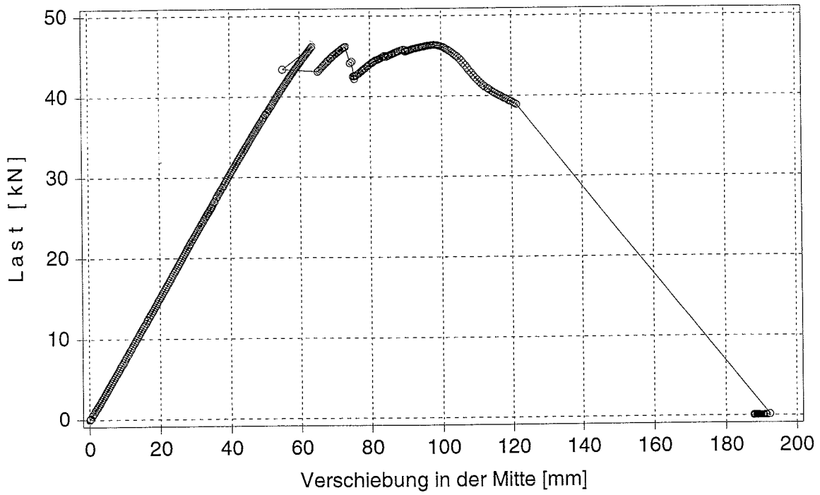
Bild C.29: Last-Verschiebungsdiagramm des Prüfkörpers KT_10_3
