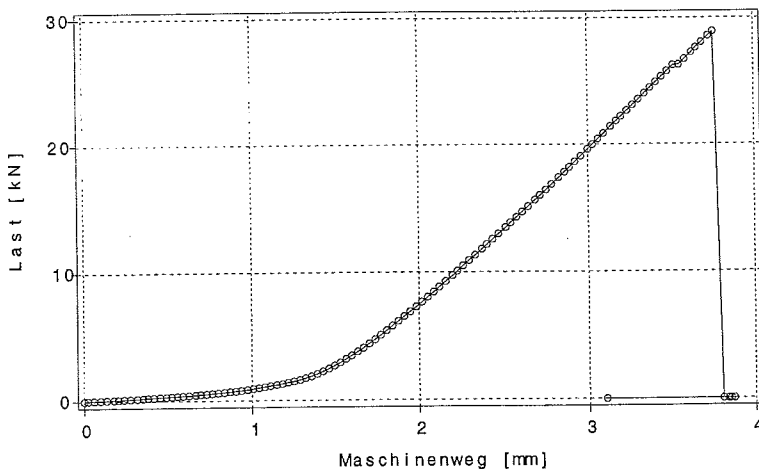
Bild B.27: Last-Verschiebungsverhalten des Prüfkörpers z2a2_2
