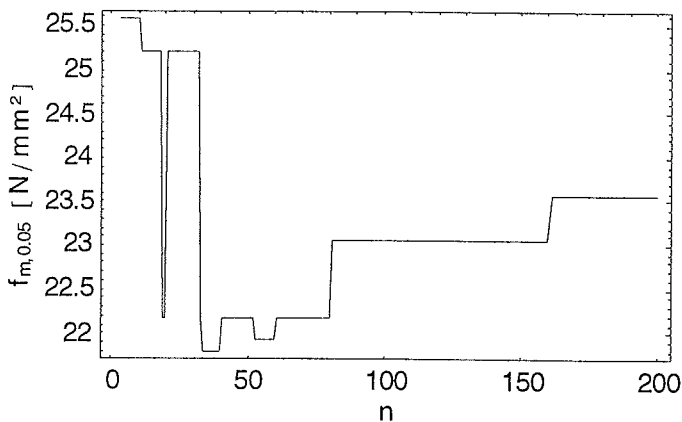
Bild 5.3.3: Zur Stabilisierung der 5%-Quantile der Biegefestigkeiten f_{m, 0.05} n = 9 , t_H = 42 mm
