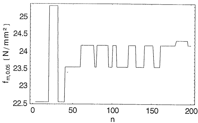
Bild 5.3.3: Zur Stabilisierung der 5%-Quantile der Biegefestigkeiten f_{m, 0.05} n = 9 , t_H = 42 mm
