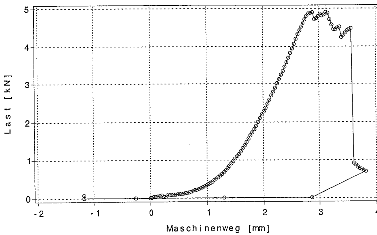
Bild B.81: Last-Verschiebungsverhalten des Prüfkörpers z3b1_1a
