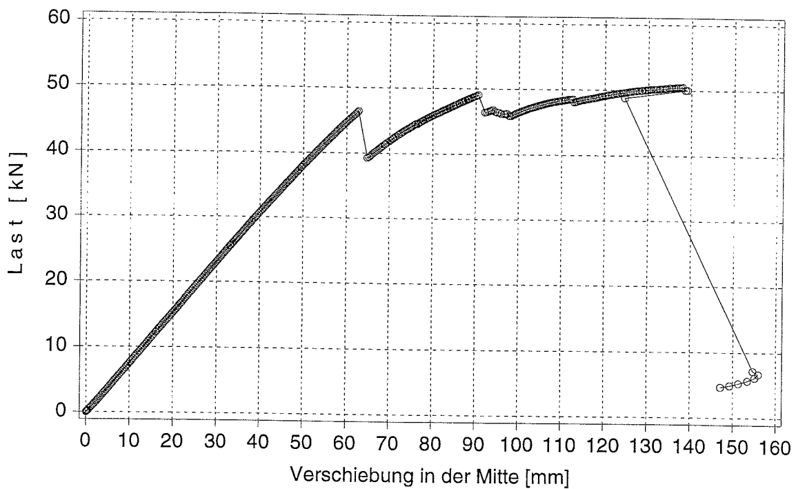
Bild C.28: Last-Verschiebungsdiagramm des Prüfkörpers KT_10_2
