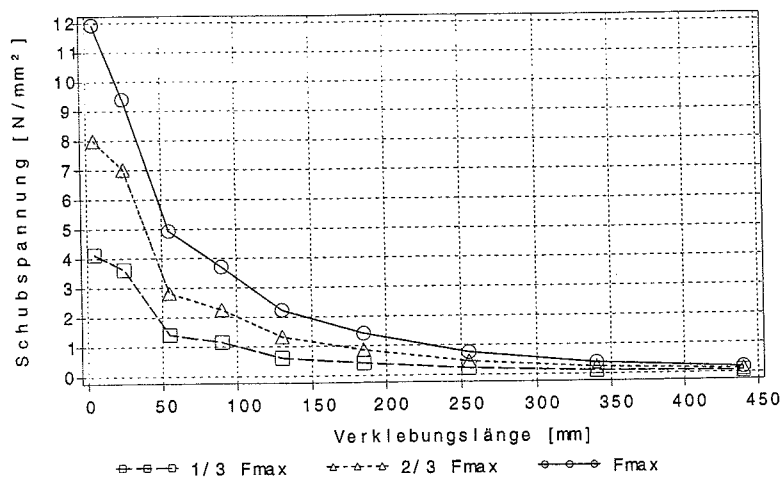
Bild B.104: Schubspannungsverläufe des Prüfkörpers z1b4_5a bei drei Laststufen
