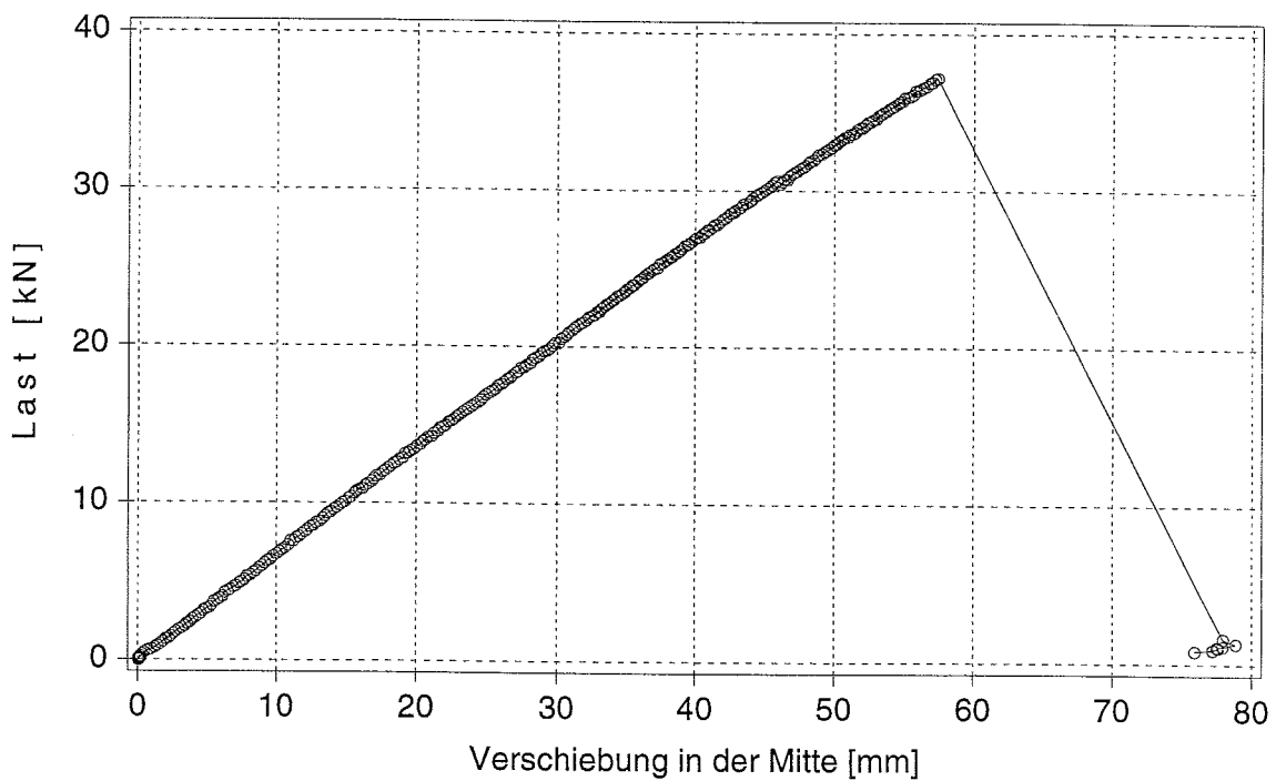
Bild C.12: Last-Verschiebungsdiagramm des Prüfkörpers KT_3_2 (T12)
