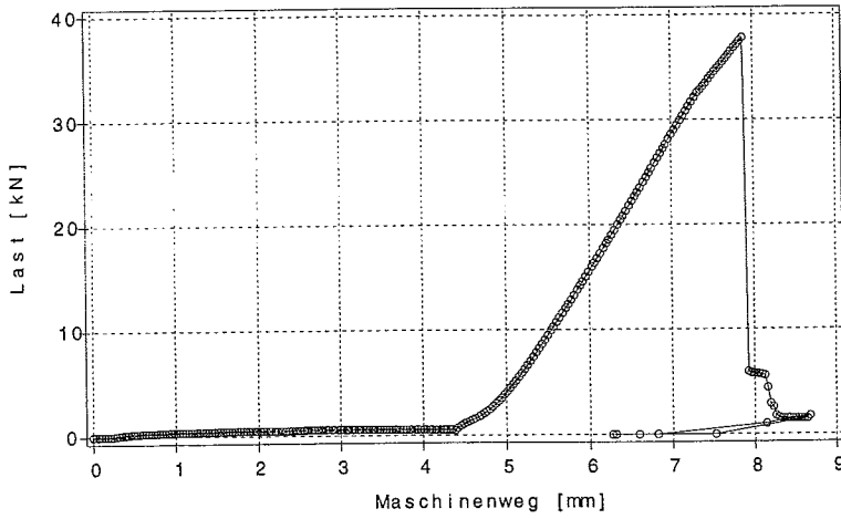
Bild B.26: Last-Verschiebungsverhalten des Prüfkörpers z2a2_1
