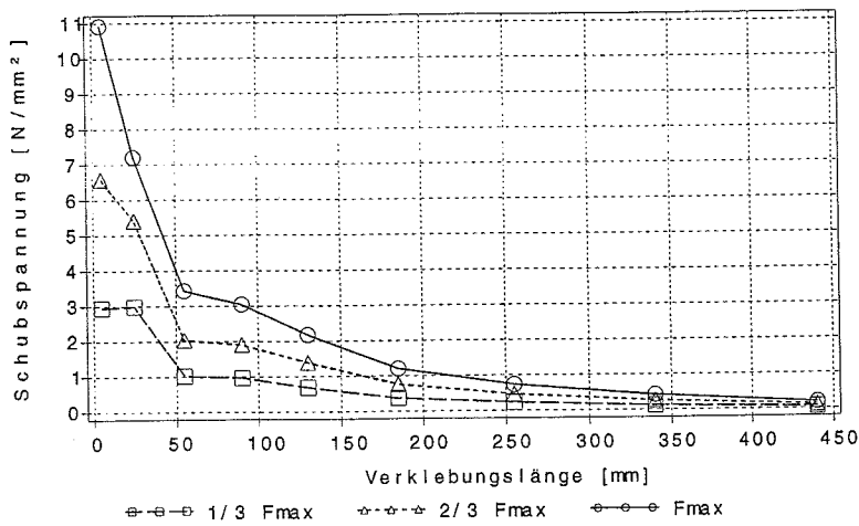
Bild B.103: Schubspannungsverläufe des Prüfkörpers z1b4_4 bei drei Laststufen
