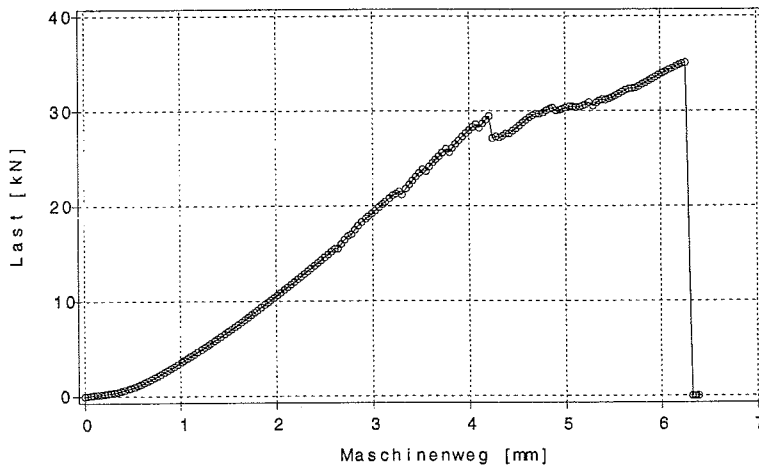
Bild B.80: Last-Verschiebungsverhalten des Prüfkörpers z3a4_5
