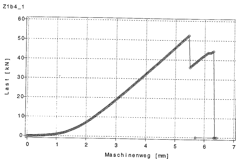
Bild B.16: Last-Verschiebungsverhalten des Prüfkörpers z1b4_1
