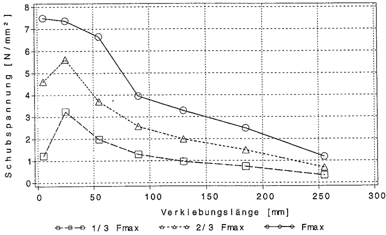
Bild B.108: Schubspannungsverläufe des Prüfkörpers z2b3_3 bei drei Laststufen
