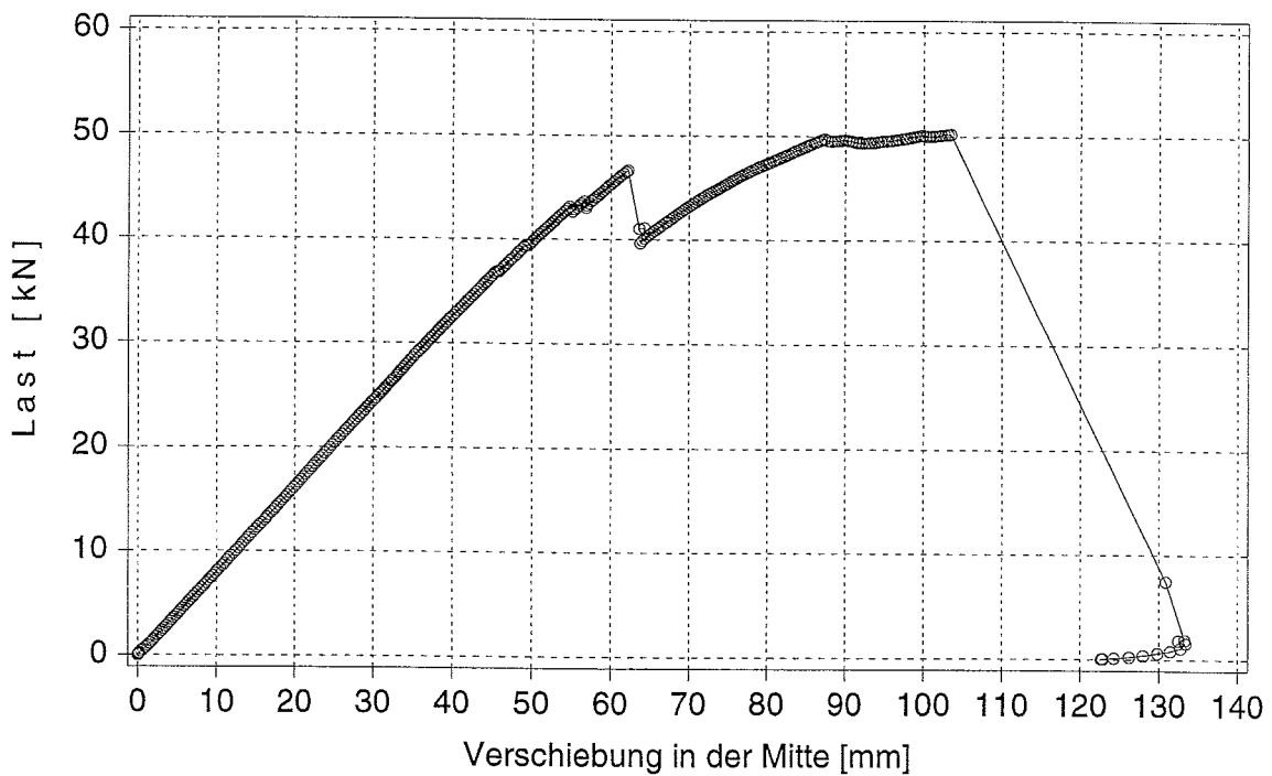
Bild C.16: Last-Verschiebungsdiagramm des Prüfkörpers KT_4_3
