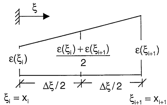
Bild 3.2.12: Angenommener Verlauf der Dehnungen zwischen zwei Dehnmessstreifen
