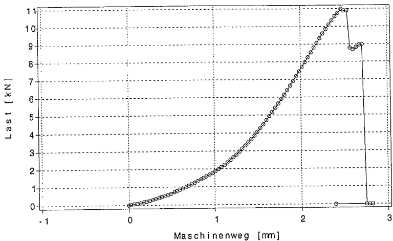
Bild B.45: Last-Verschiebungsverhalten des Prüfkörpers z2b1_5
