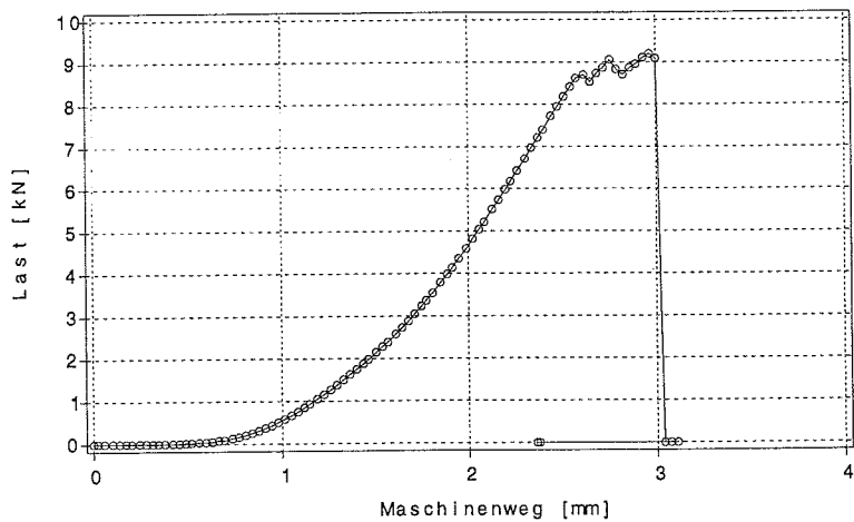
Bild B.44: Last-Verschiebungsverhalten des Prüfkörpers z2b1_4
