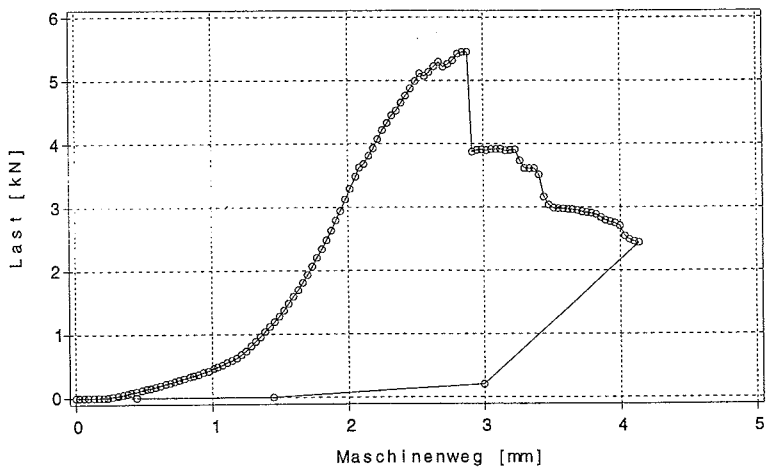
Bild B.43: Last-Verschiebungsverhalten des Prüfkörpers z2b1_3
