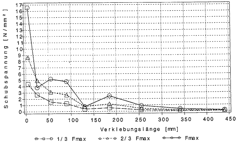
Bild B.102: Schubspannungsverläufe des Prüfkörpers z1b4_3 bei drei Laststufen
