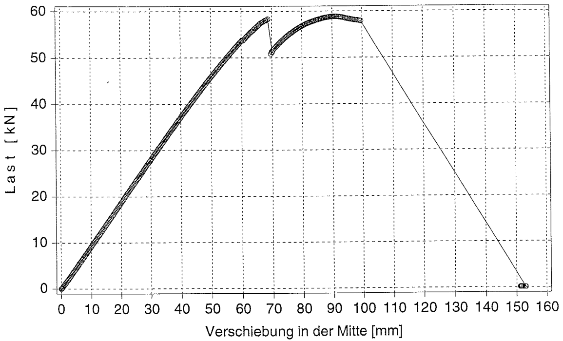
Bild C.17: Last-Verschiebungsdiagramm des Prüfkörpers KT_5_1
