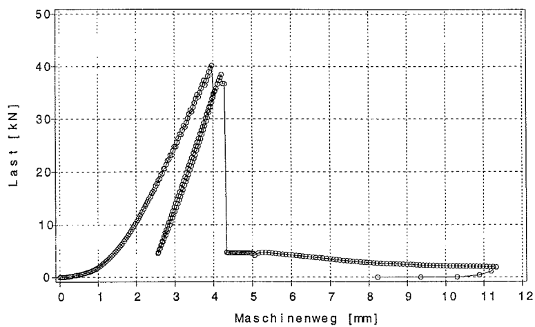
Bild B.60: Last-Verschiebungsverhalten des Prüfkörpers z2b4_5
