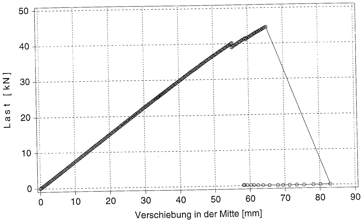
Bild C.34: Last-Verschiebungsdiagramm des Prüfkörpers KT_11_5
