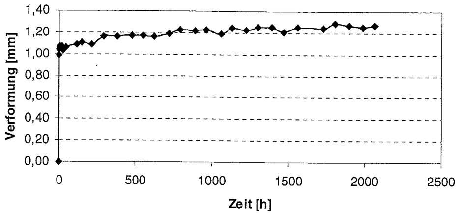
Bild 6.6: Mittelwert der Verformungen im querkraftfreien Bereich des Trägers LT_1
