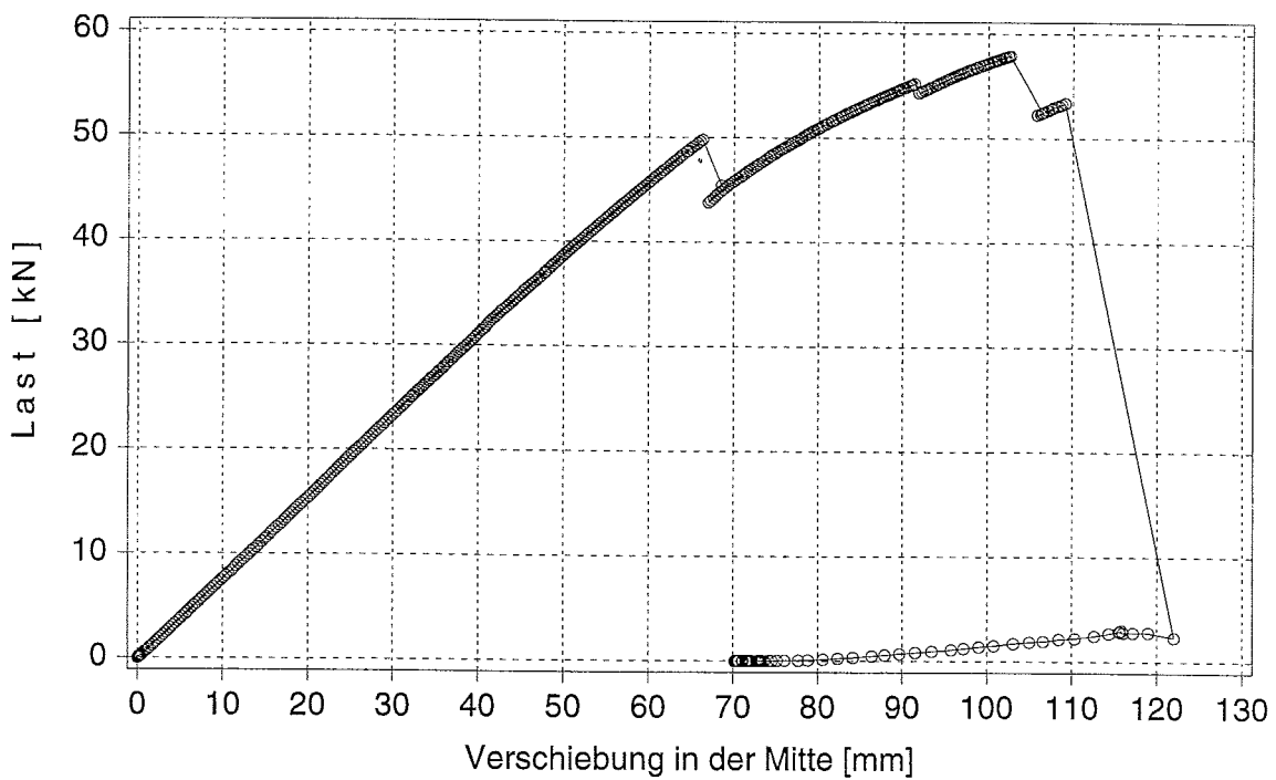
Bild C.20: Last-Verschiebungsdiagramm des Prüfkörpers KT_5_4
