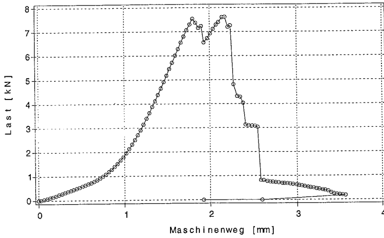
Bild B.25: Last-Verschiebungsverhalten des Prüfkörpers z2a1_5
