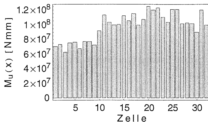
Bild 5.2.6: Aufnehmbare Biegemomente
