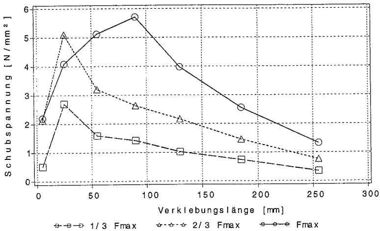
Bild B.109: Schubspannungsverläufe des Prüfkörpers z2b3_4 bei drei Laststufen
