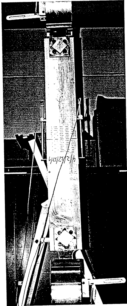
Bild A-10: Versuchsaufbau der Prüfkörperform 2
