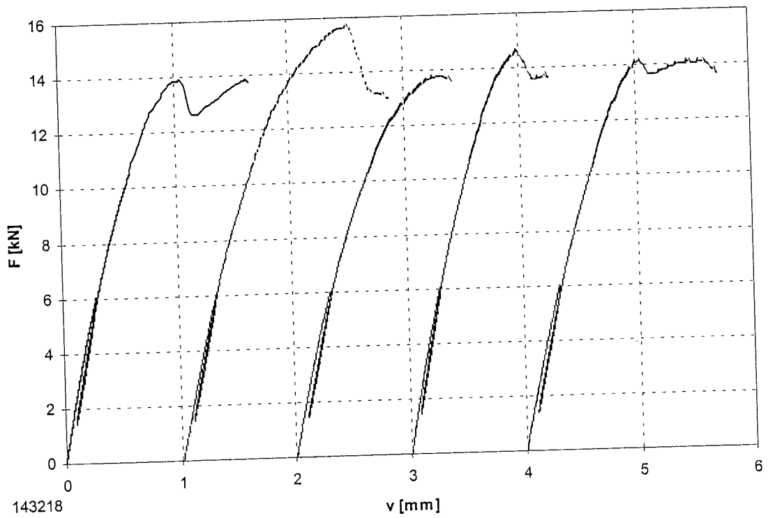
Bild B-68: Last-Verschiebungsdiagramm der Versuchsreihe 143218
