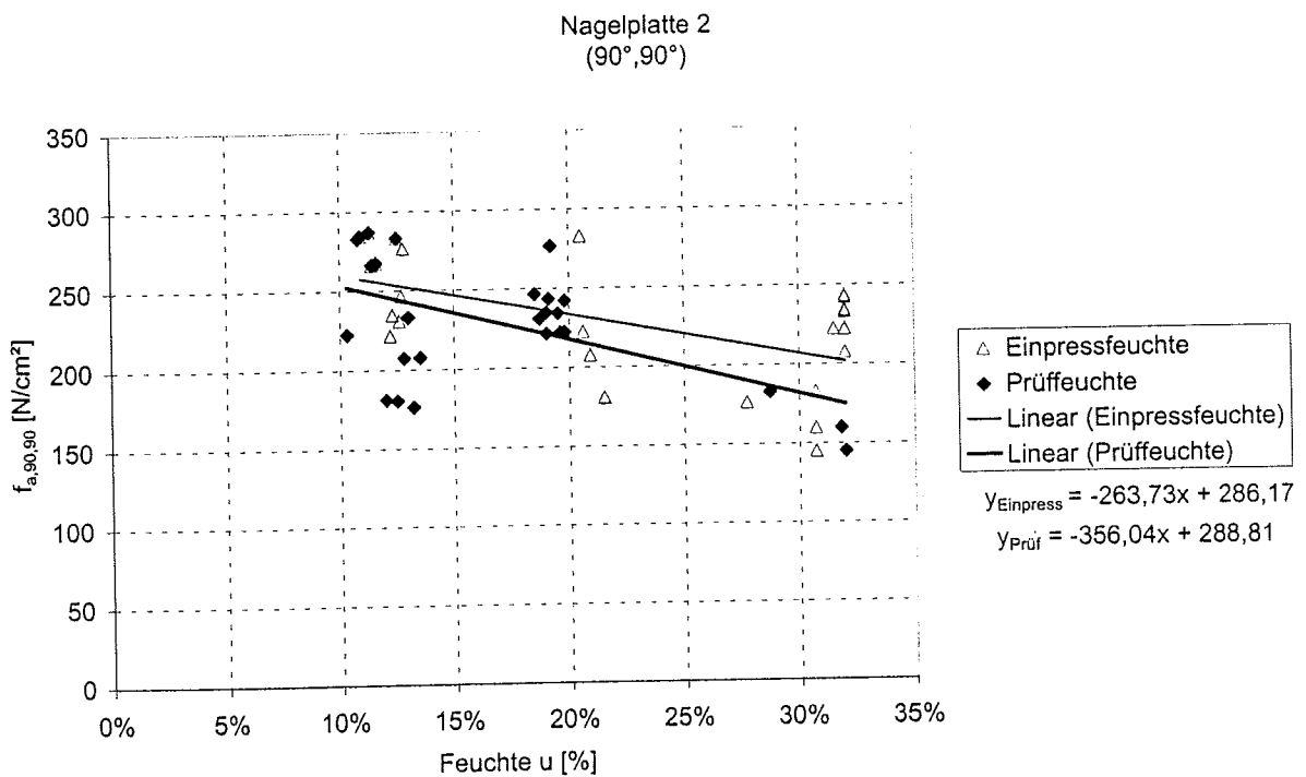
Bild C-24: Einzelwerte der Verankerungsfestigkeit mit der Einpress- bzw. Prüffeuchte, Nagelplatte 2, Winkelkombination 4
