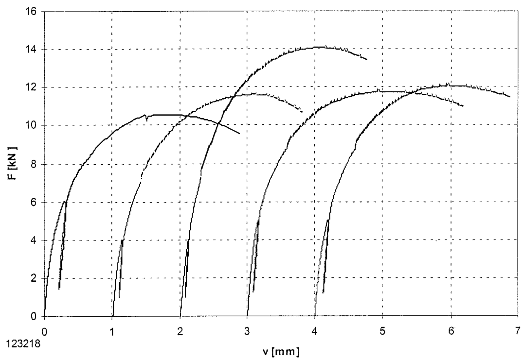
Bild B-66: Last-Verschiebungsdiagramm der Versuchsreihe 123218
