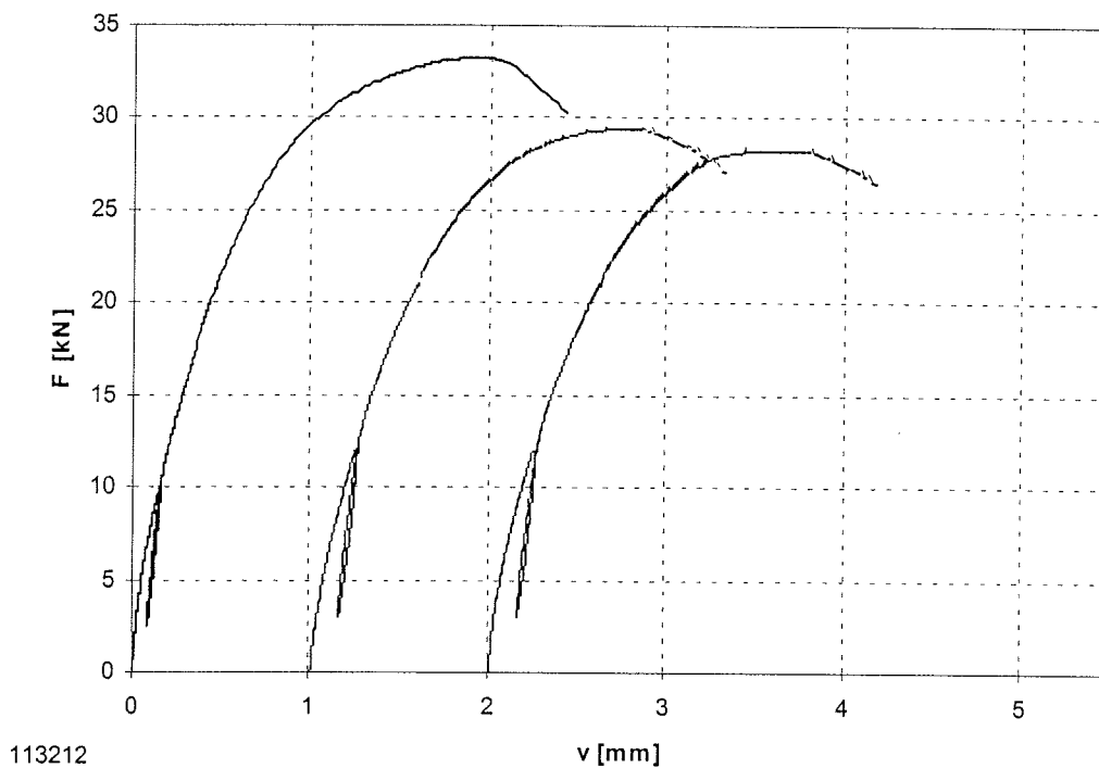
Bild B-33: Last-Verschiebungsdiagramm der Versuchsreihe 113212
