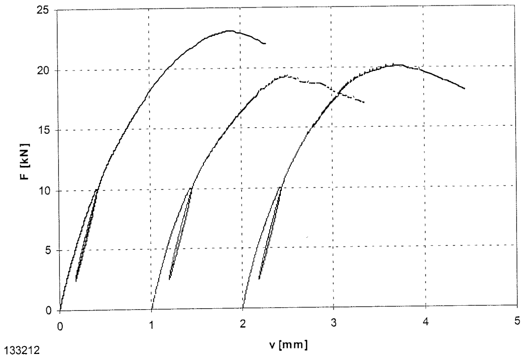
Bild B-35: Last-Verschiebungsdiagramm der Versuchsreihe 133212
