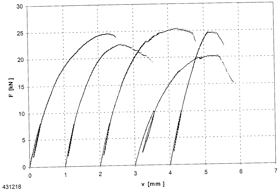
Bild B-63: Last-Verschiebungsdiagramm der Versuchsreihe 431218
