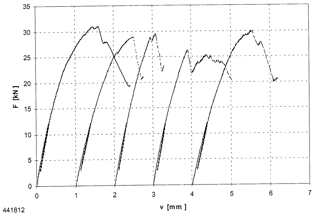
Bild B-32: Last-Verschiebungsdiagramm der Versuchsreihe 441812
