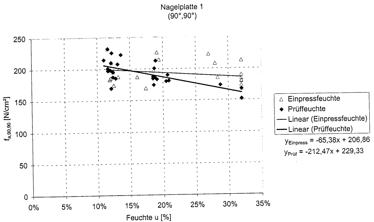
Bild C-20: Einzelwerte der Verankerungsfestigkeit mit der Einpress- bzw. Prüffeuchte, Nagelplatte 1, Winkelkombination 4
