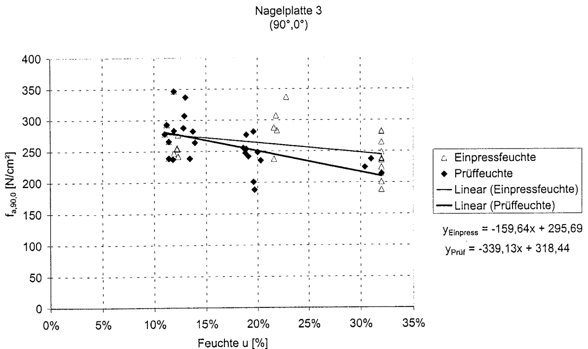
Bild C-26: Einzelwerte der Verankerungsfestigkeit mit der Einpress- bzw. Prüffeuchte, Nagelplatte 3, Winkelkombination 2
