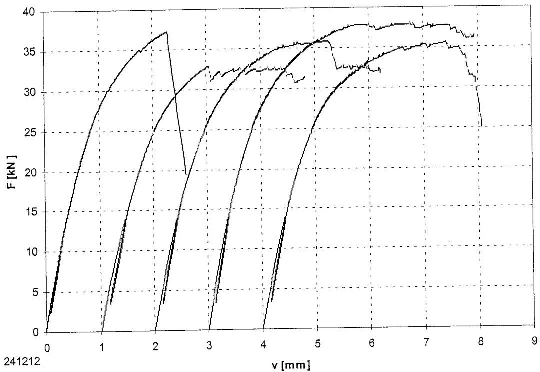
Bild B-8: Last-Verschiebungsdiagramm der Versuchsreihe 241212 (Biegebruch bei allen Prüfkörpern)
