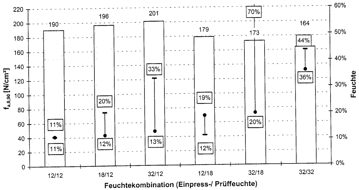
Bild C-11: Mittelwerte der Verankerungsfestigkeit, der Einpress- und Prüffeuchte der Nagelplatte 3 mit Winkelkombination 3
