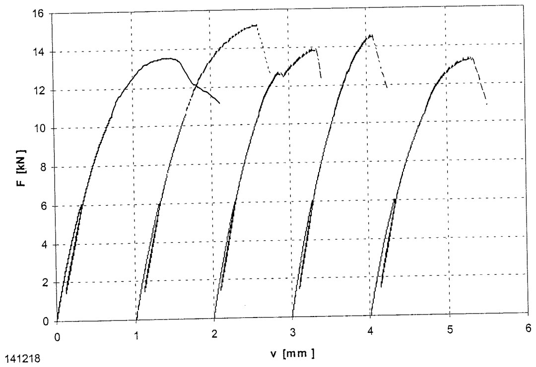
Bild B-52: Last-Verschiebungsdiagramm der Versuchsreihe 141218
