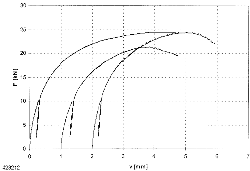
Bild B-46: Last-Verschiebungsdiagramm der Versuchsreihe 423212
