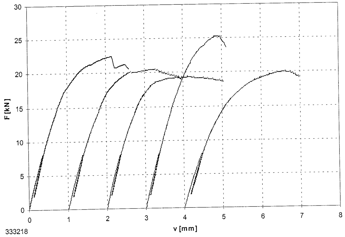
Bild B-75: Last-Verschiebungsdiagramm der Versuchsreihe 333218
