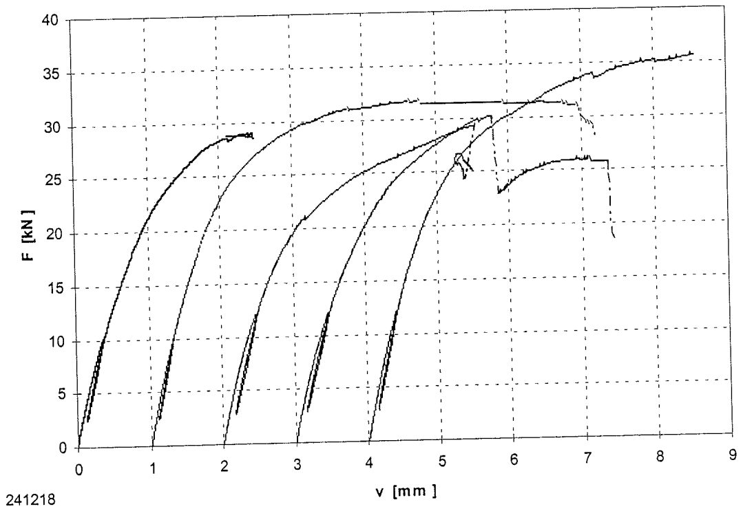
Bild B-56: Last-Verschiebungsdiagramm der Versuchsreihe 241218
