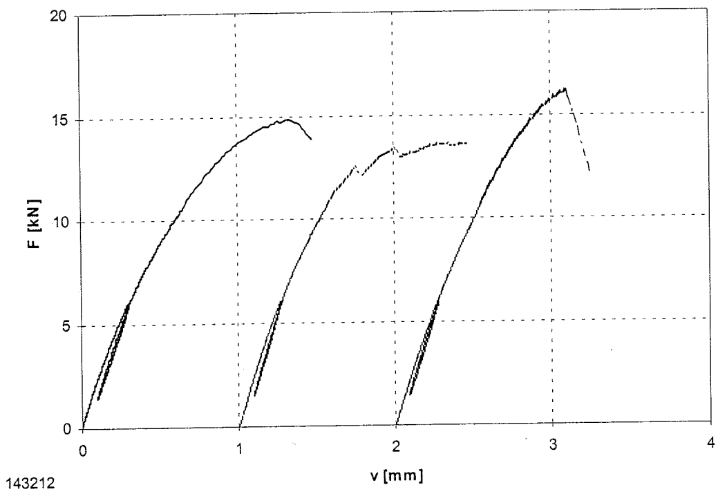
Bild B-36: Last-Verschiebungsdiagramm der Versuchsreihe 143212
