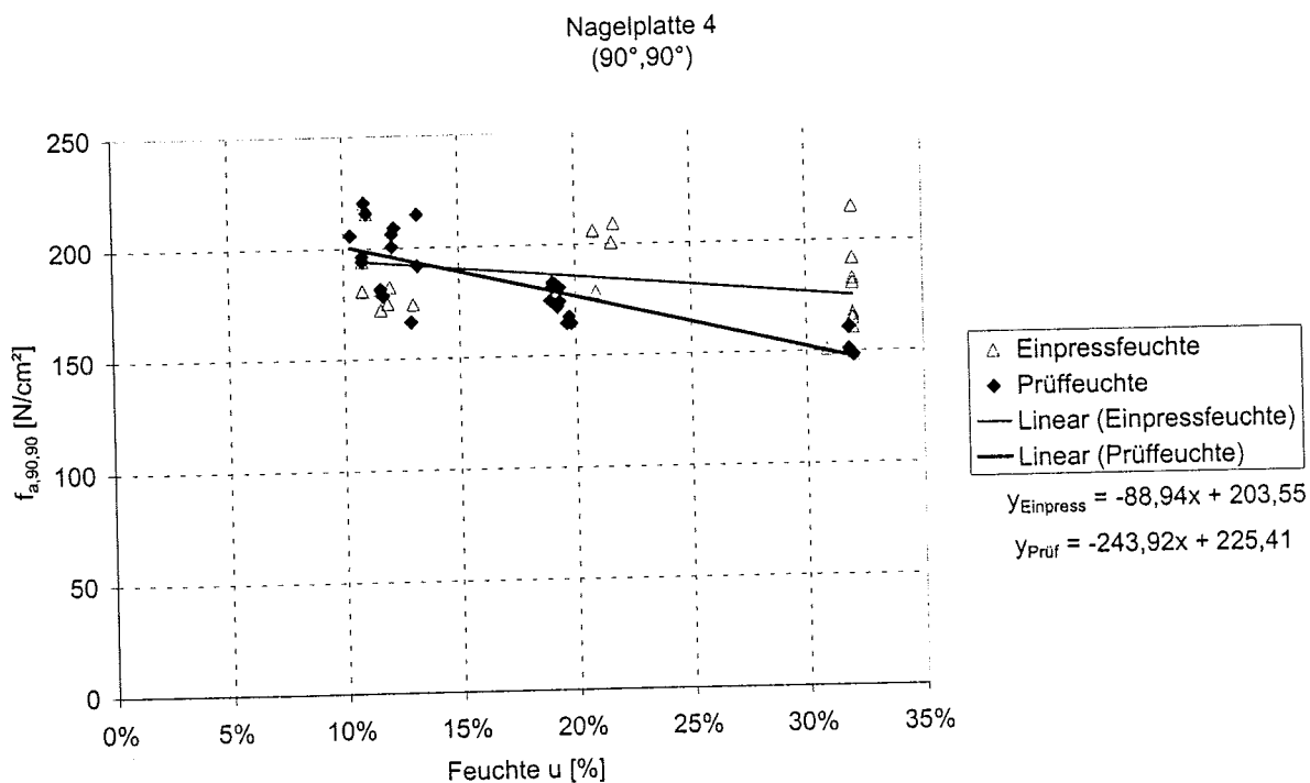
Bild C-32: Einzelwerte der Verankerungsfestigkeit mit der Einpress- bzw. Prüffeuchte, Nagelplatte 4, Winkelkombination 4
