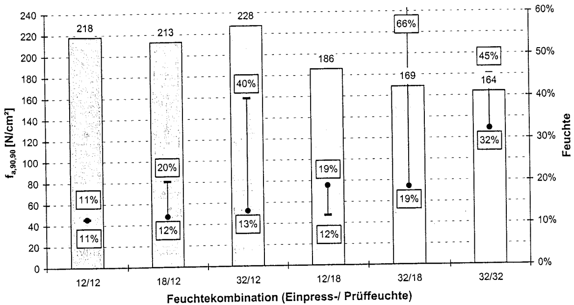
Bild C-12: Mittelwerte der Verankerungsfestigkeit, der Einpress- und Prüffeuchte der Nagelplatte 3 mit Winkelkombination 4
