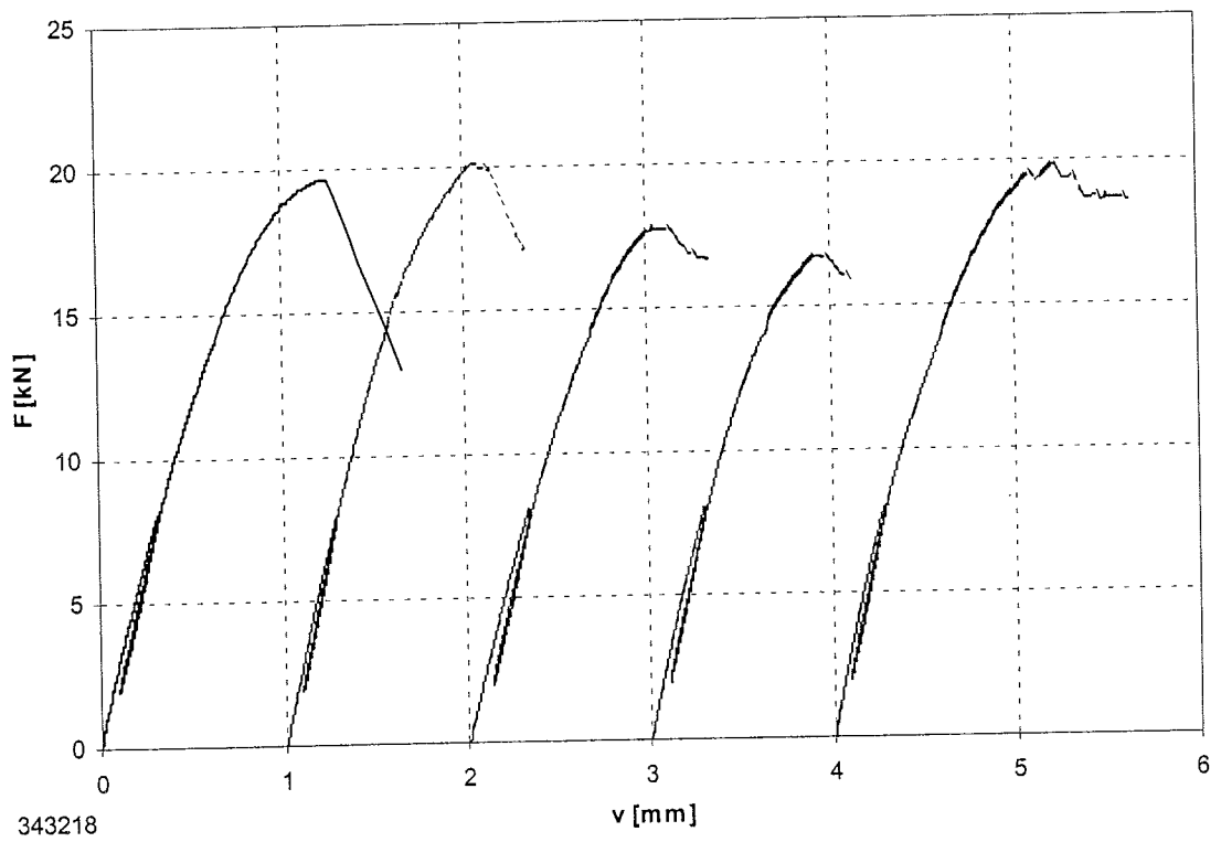
Bild B-76: Last-Verschiebungsdiagramm der Versuchsreihe 343218
