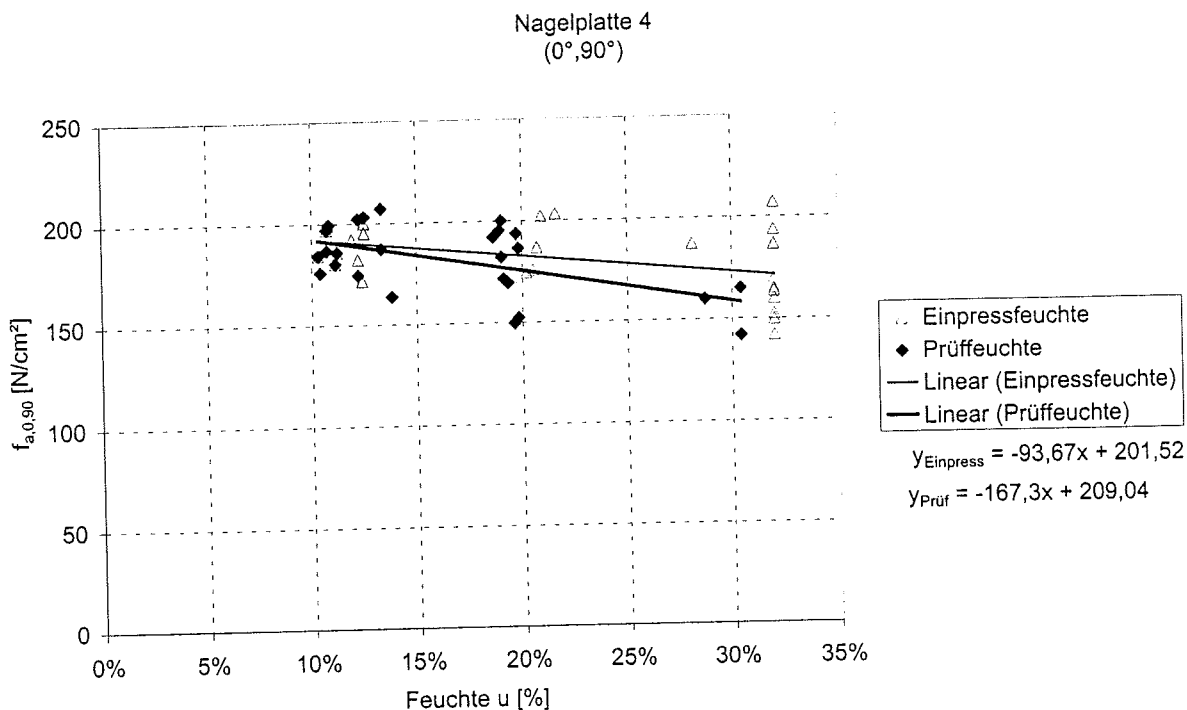
Bild C-31: Einzelwerte der Verankerungsfestigkeit mit der Einpress- bzw. Prüffeuchte, Nagelplatte 4, Winkelkombination 3
