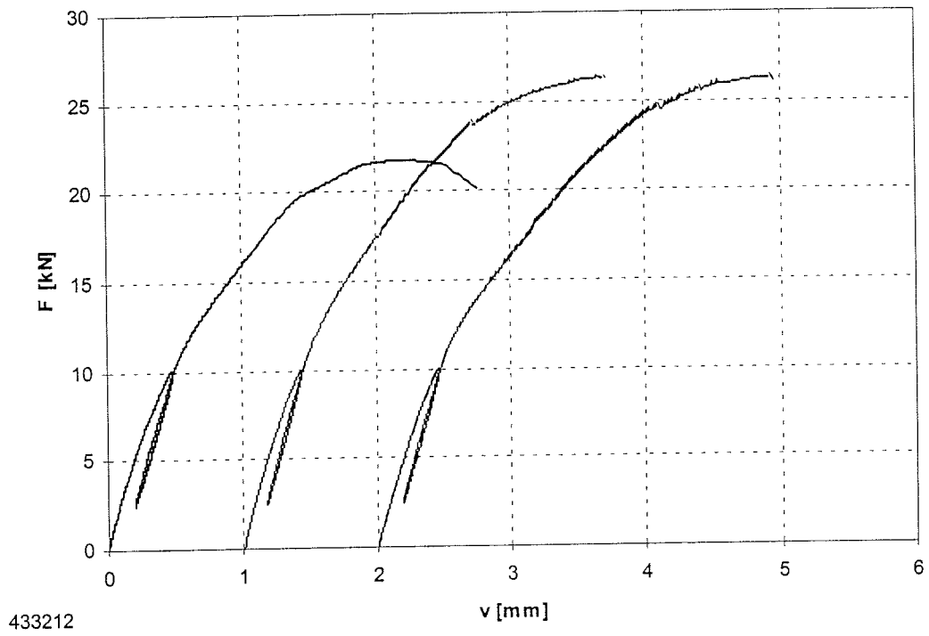
Bild B-47: Last-Verschiebungsdiagramm der Versuchsreihe 433212
