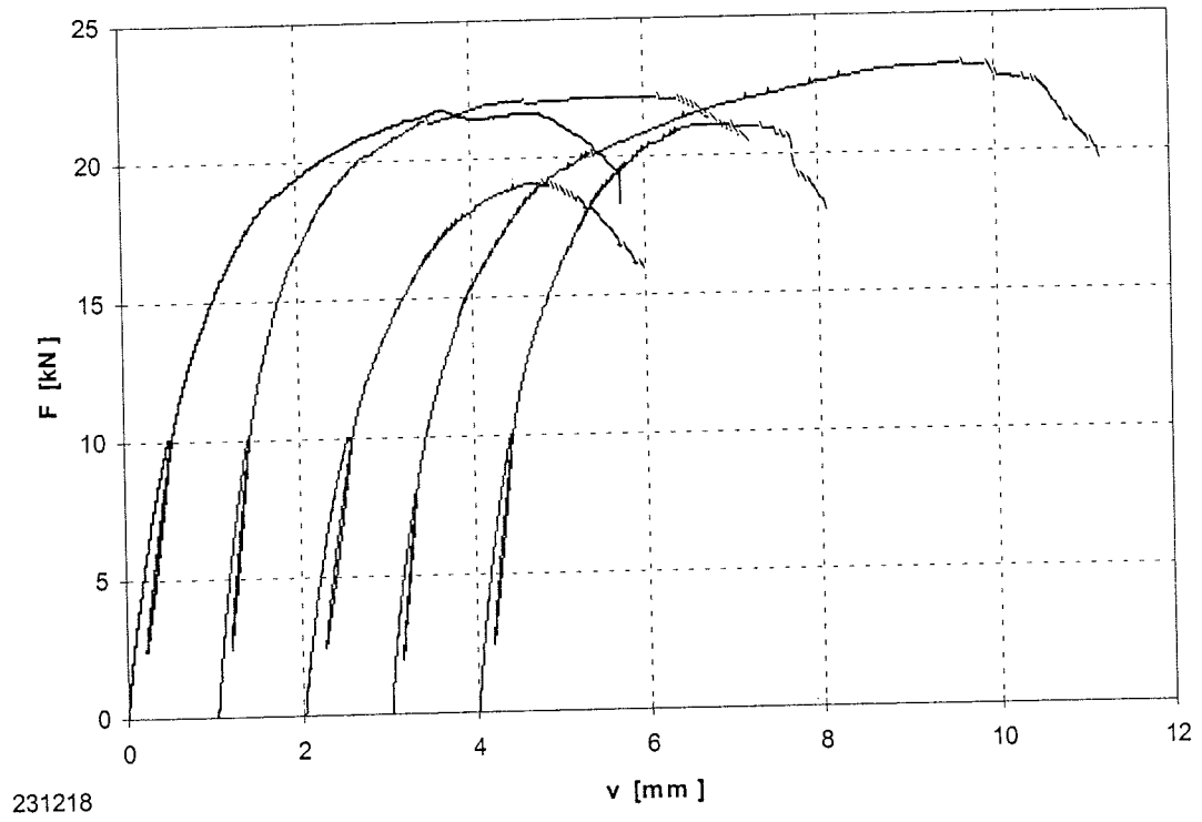
Bild B-55: Last-Verschiebungsdiagramm der Versuchsreihe 231218
