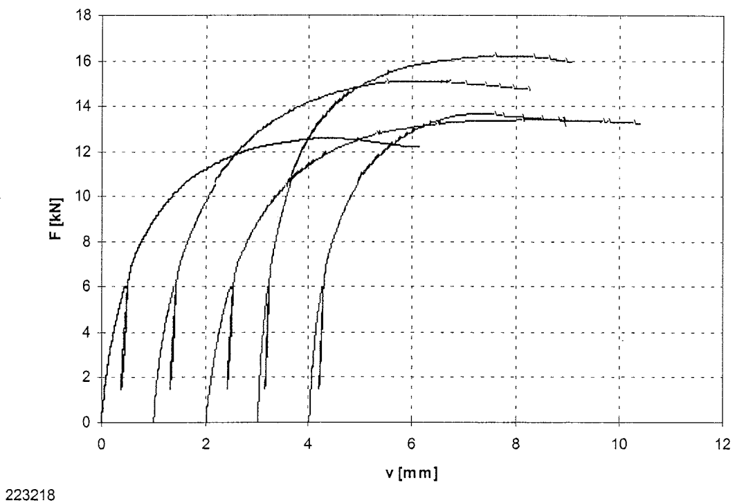
Bild B-70: Last-Verschiebungsdiagramm der Versuchsreihe 223218
