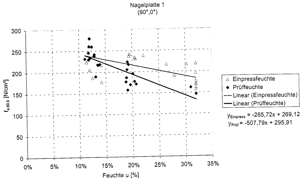
Bild 5: Beispiel für einen Einfluss der Einpress- und Prüffeuchte auf die Verankerungsfestigkeit
