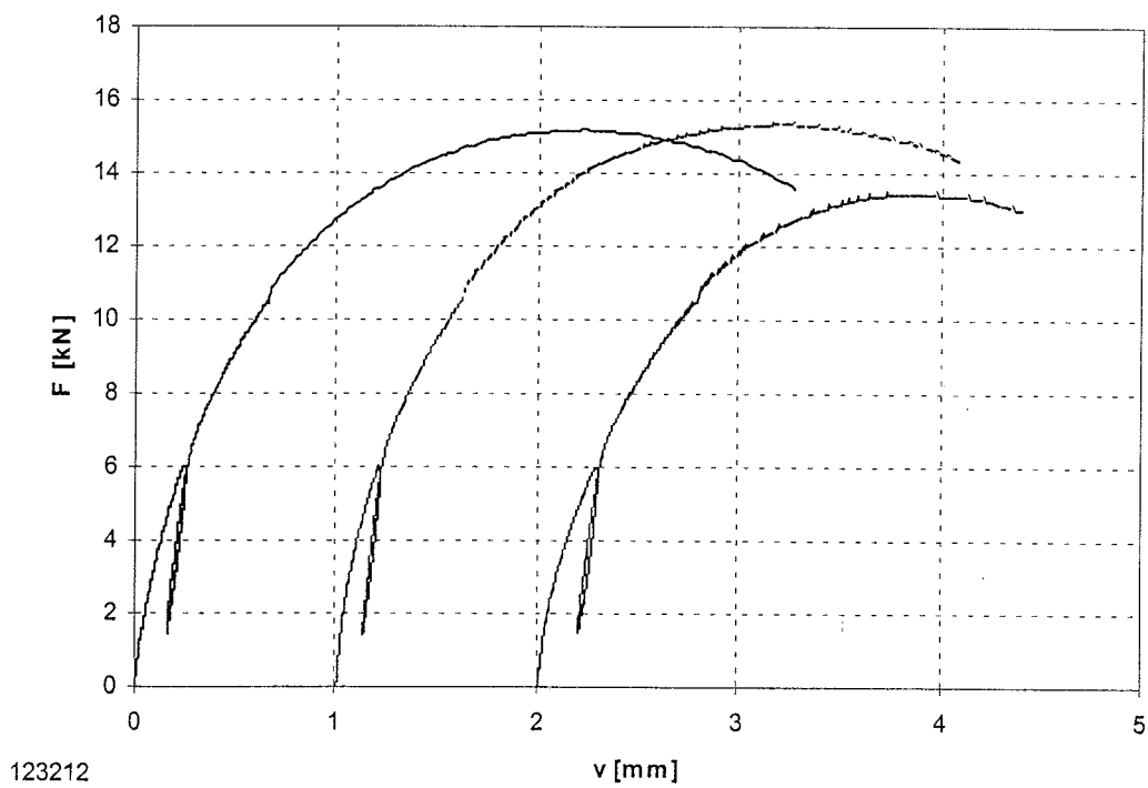
Bild B-34: Last-Verschiebungsdiagramm der Versuchsreihe 123212
