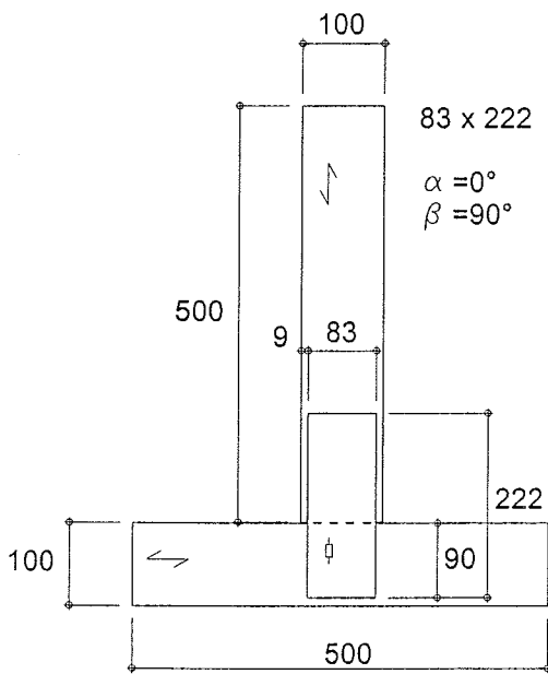
Bild A-5: Prüfkörper der Nagelplatte 1 – Form und Maße
