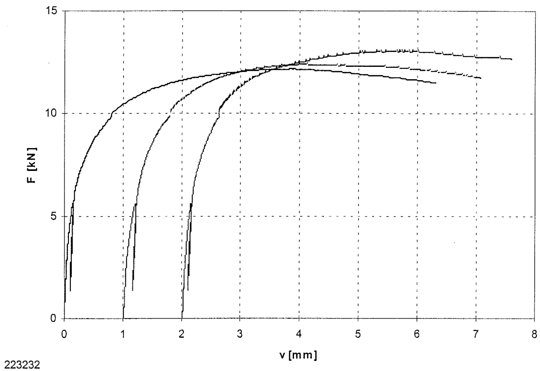
Bild B-86: Last-Verschiebungsdiagramm der Versuchsreihe 223232
