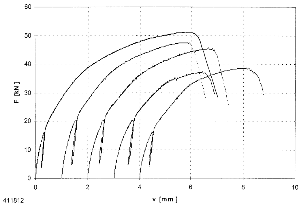
Bild B-29: Last-Verschiebungsdiagramm der Versuchsreihe 411812
