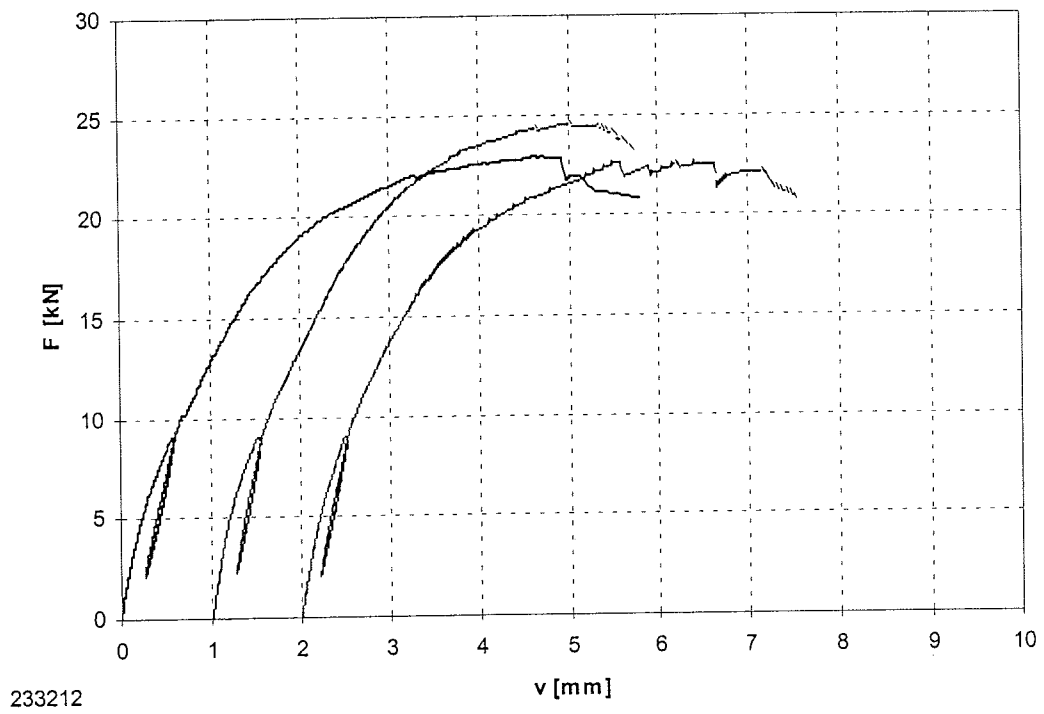
Bild B-39: Last-Verschiebungsdiagramm der Versuchsreihe 233212
