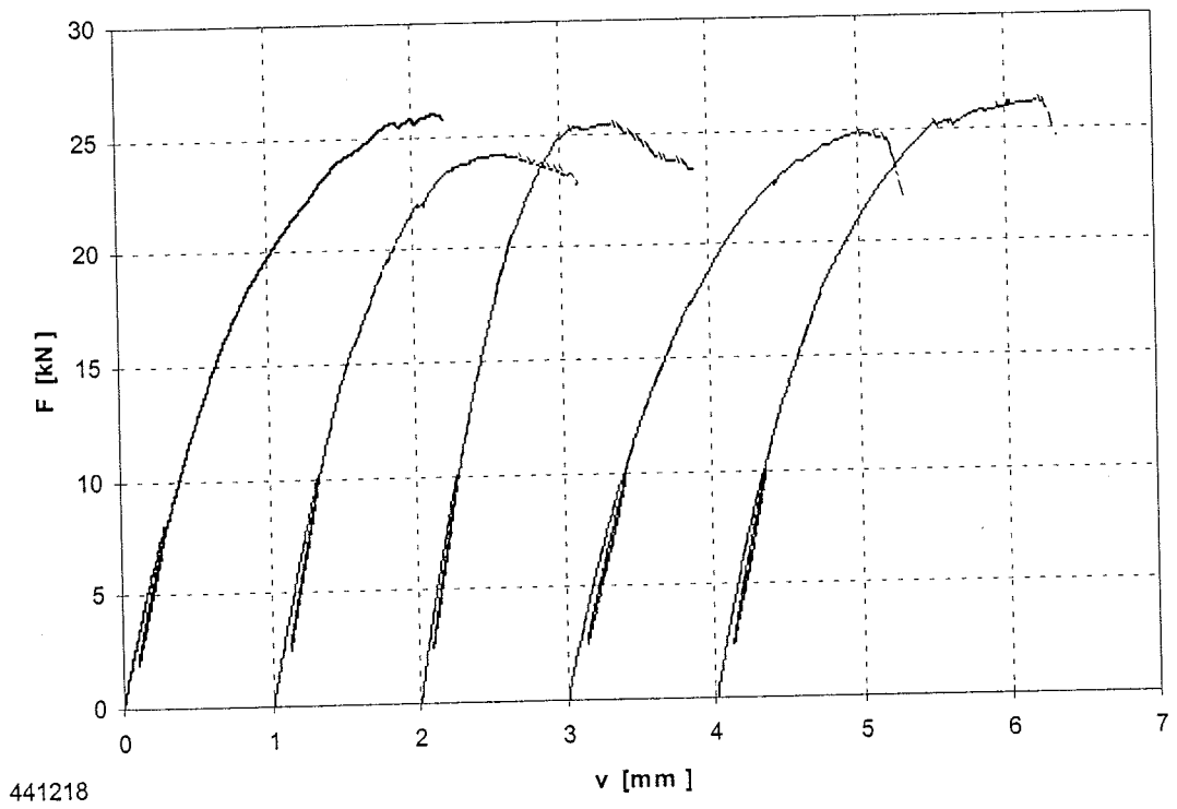
Bild B-64: Last-Verschiebungsdiagramm der Versuchsreihe 441218
