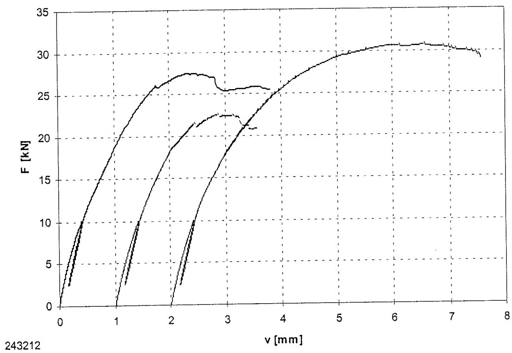
Bild B-40: Last-Verschiebungsdiagramm der Versuchsreihe 243212
