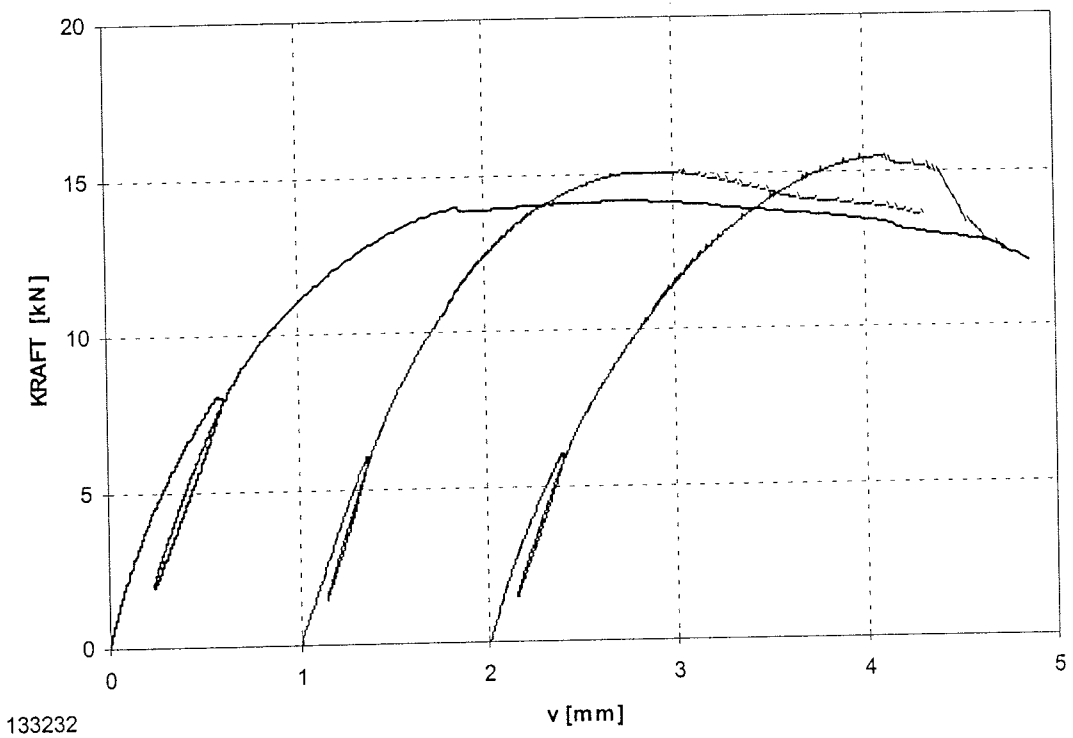
Bild B-83: Last-Verschiebungsdiagramm der Versuchsreihe 133232
