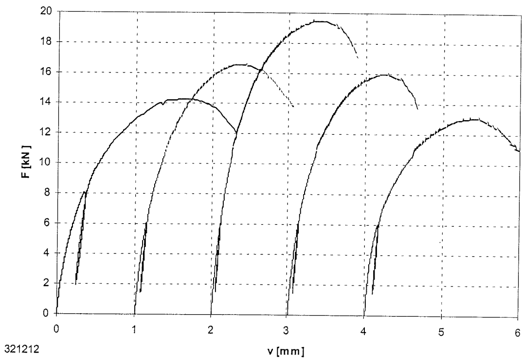
Bild B-10: Last-Verschiebungsdiagramm der Versuchsreihe 321212
