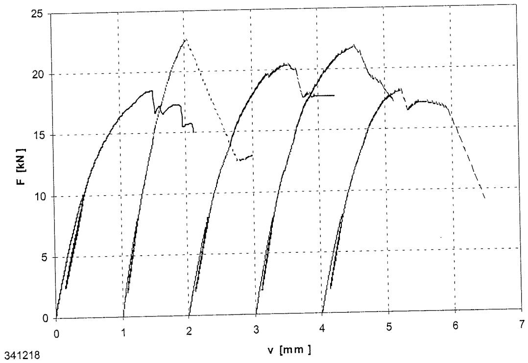
Bild B-60: Last-Verschiebungsdiagramm der Versuchsreihe 341218
