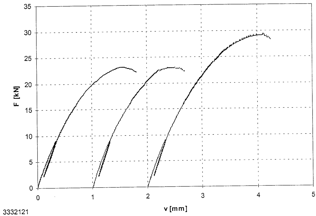
Bild B-43: Last-Verschiebungsdiagramm der Versuchsreihe 333212
