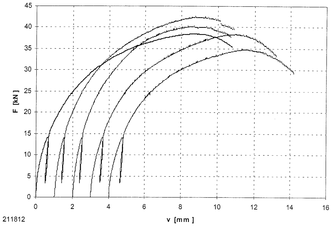
Bild B-21: Last-Verschiebungsdiagramm der Versuchsreihe 211812
