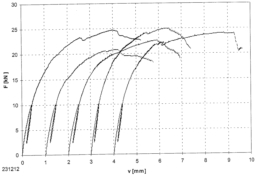
Bild B-7: Last-Verschiebungsdiagramm der Versuchsreihe 231212
