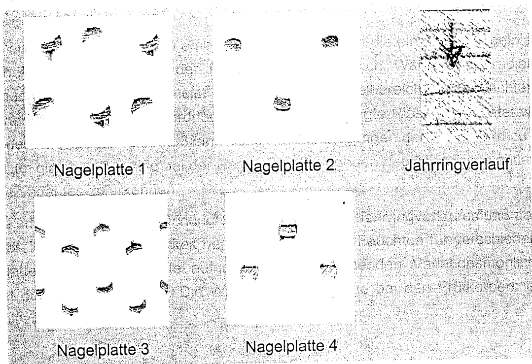
Bild 2: Eingepresste Nägel der einzelnen Nagelplatten (unbelastet) – radial
