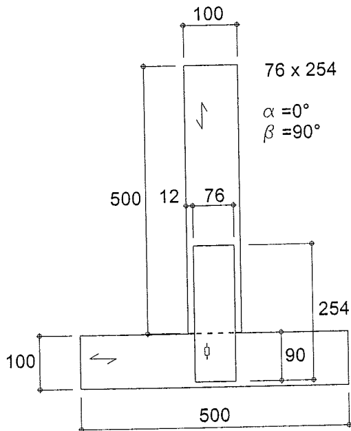
Bild A-8: Prüfkörper der Nagelplatte 4 – Form und Maße
