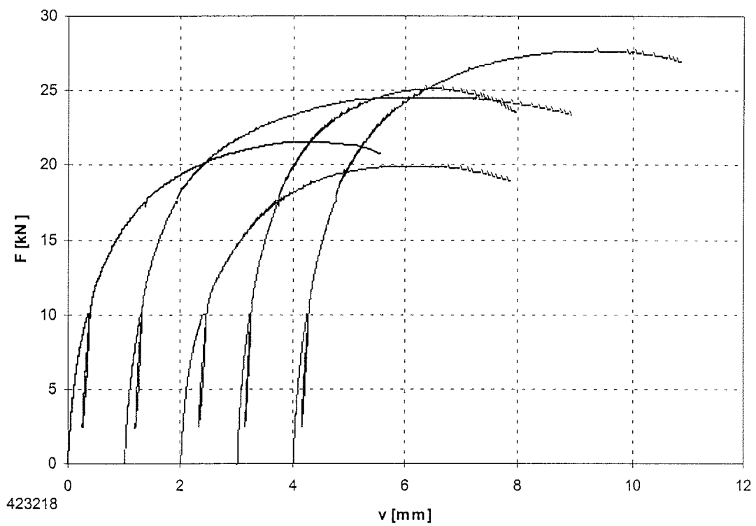
Bild B-78: Last-Verschiebungsdiagramm der Versuchsreihe 423218
