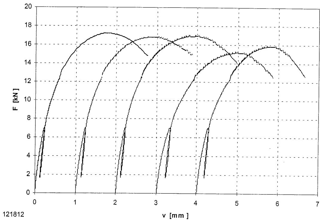
Bild B-18: Last-Verschiebungsdiagramm der Versuchsreihe 121812
