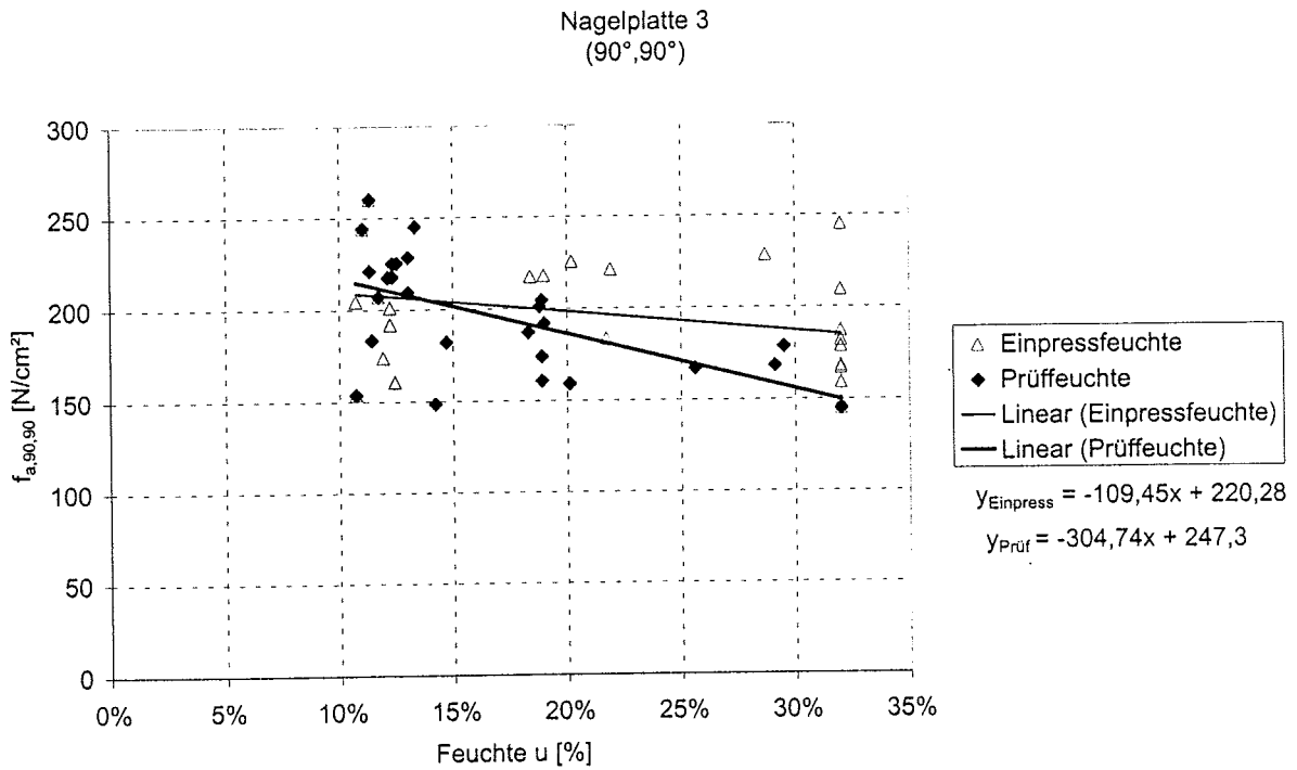
Bild C-28: Einzelwerte der Verankerungsfestigkeit mit der Einpress- bzw. Prüffeuchte, Nagelplatte 3, Winkelkombination 4
