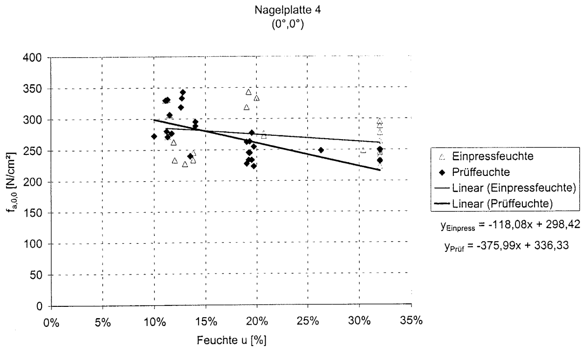
Bild C-29: Einzelwerte der Verankerungsfestigkeit mit der Einpress- bzw. Prüffeuchte, Nagelplatte 4, Winkelkombination 1
