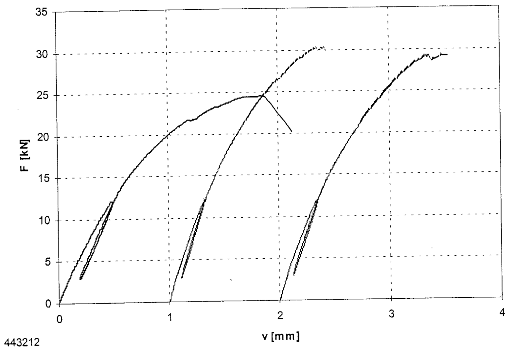
Bild B-48: Last-Verschiebungsdiagramm der Versuchsreihe 443212
