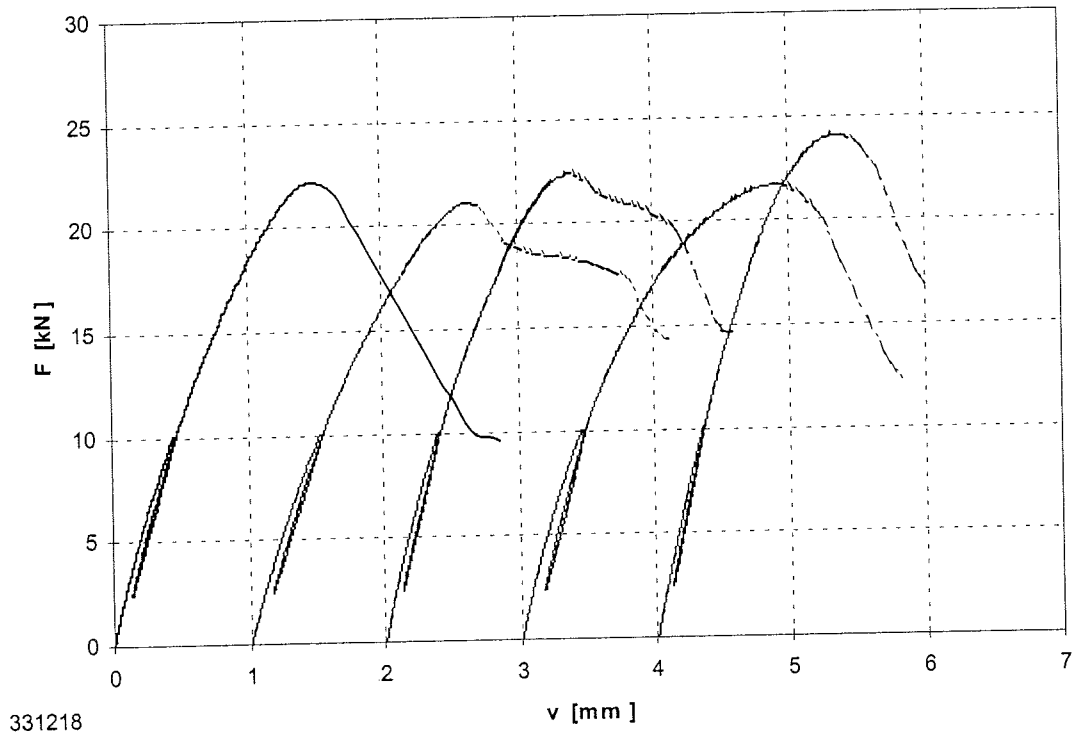
Bild B-59: Last-Verschiebungsdiagramm der Versuchsreihe 331218
