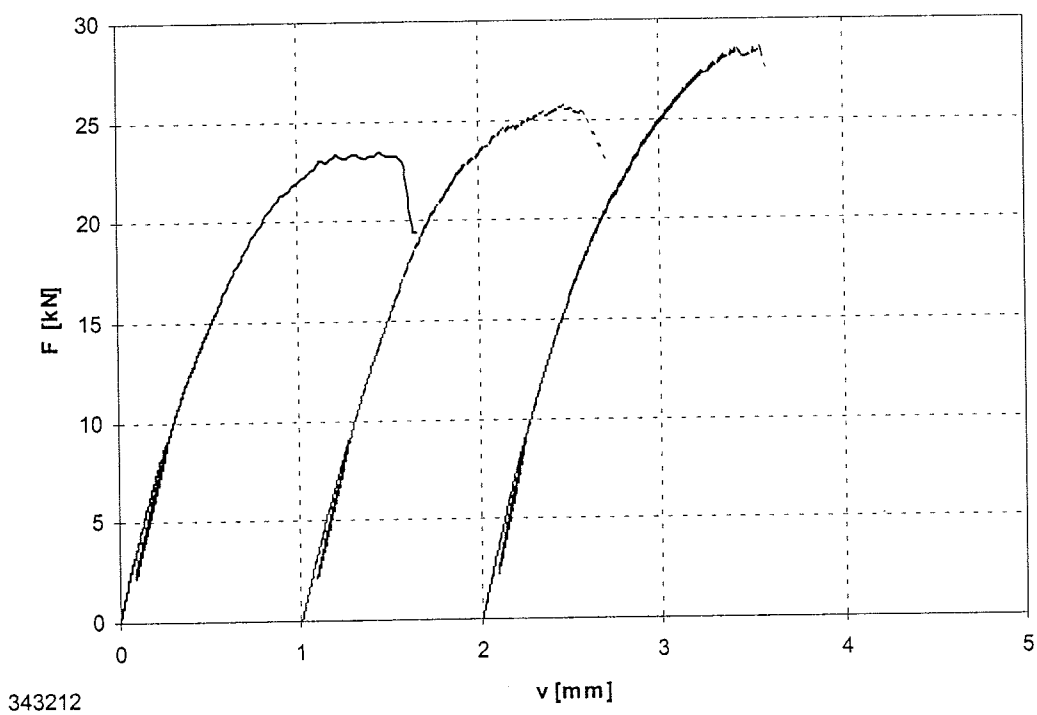
Bild B-44: Last-Verschiebungsdiagramm der Versuchsreihe 343212
