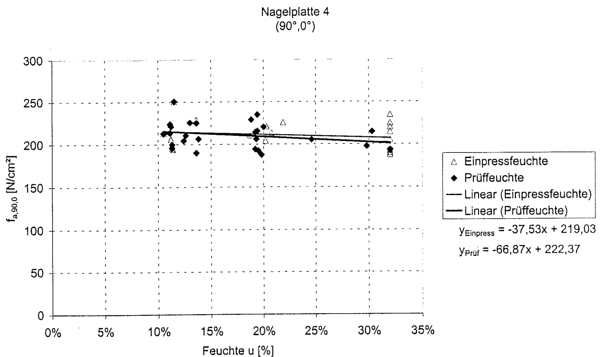
Bild C-30: Einzelwerte der Verankerungsfestigkeit mit der Einpress- bzw. Prüffeuchte, Nagelplatte 4, Winkelkombination 2
