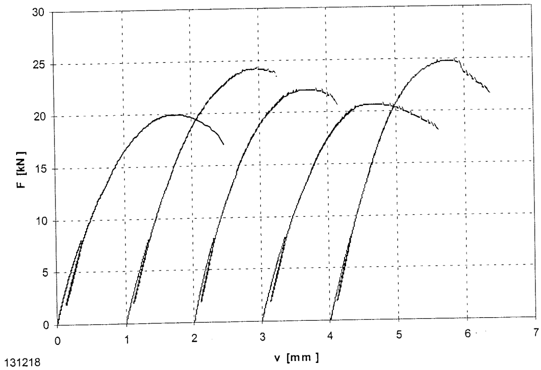
Bild B-51: Last-Verschiebungsdiagramm der Versuchsreihe 131218
