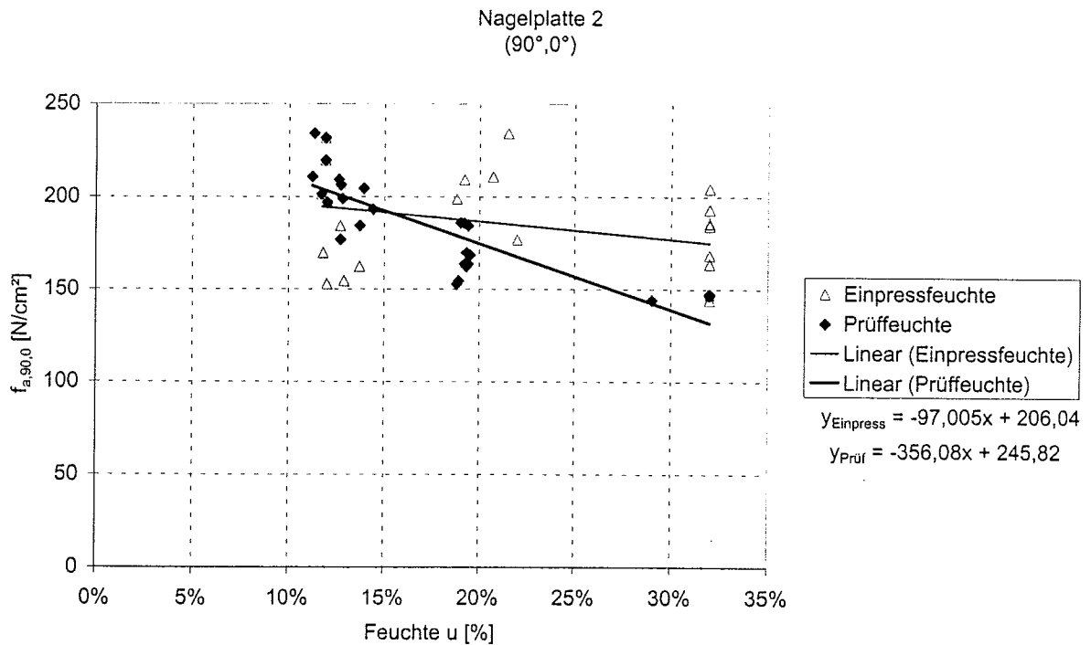
Bild C-22: Einzelwerte der Verankerungsfestigkeit mit der Einpress- bzw. Prüffeuchte, Nagelplatte 2, Winkelkombination 2
