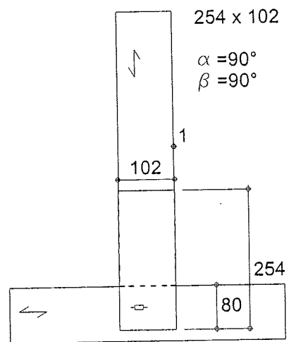
Bild A-8: Prüfkörper der Nagelplatte 4 – Form und Maße
