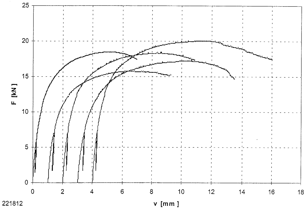
Bild B-22: Last-Verschiebungsdiagramm der Versuchsreihe 221812
