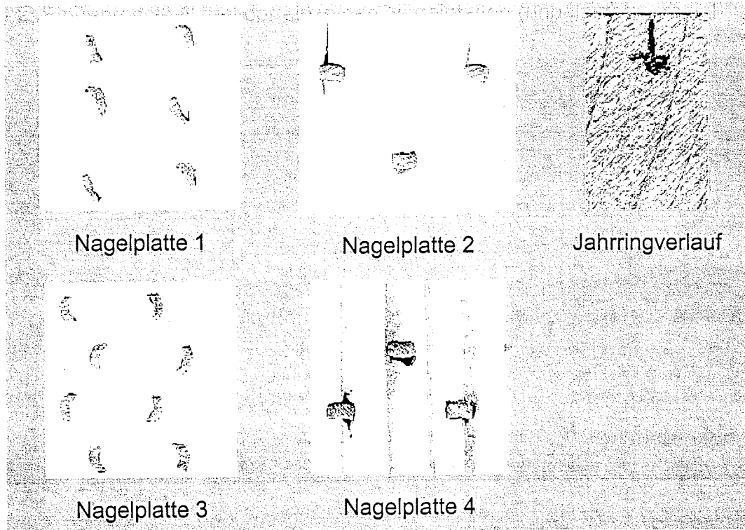
Bild 3: Eingepresste Nägel der einzelnen Nagelplatten (unbelastet) - tangential
