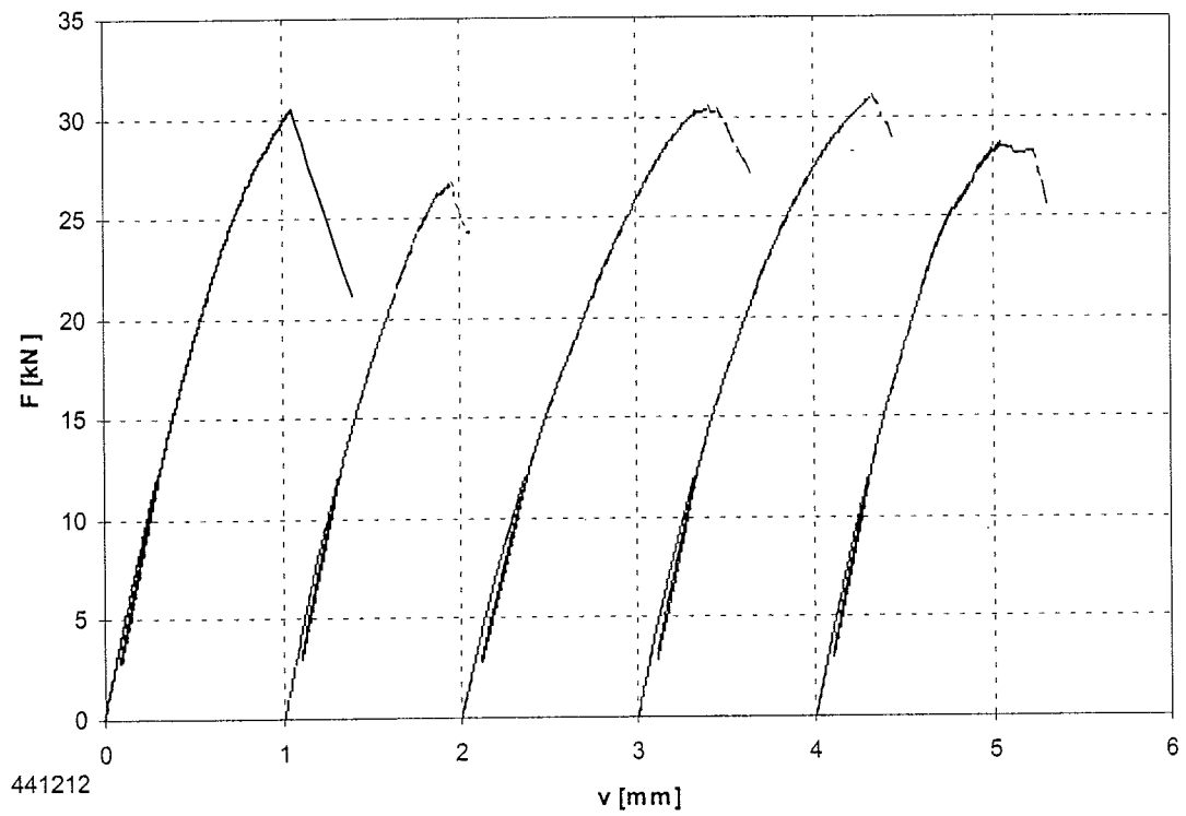
Bild B-16: Last-Verschiebungsdiagramm der Versuchsreihe 441212
