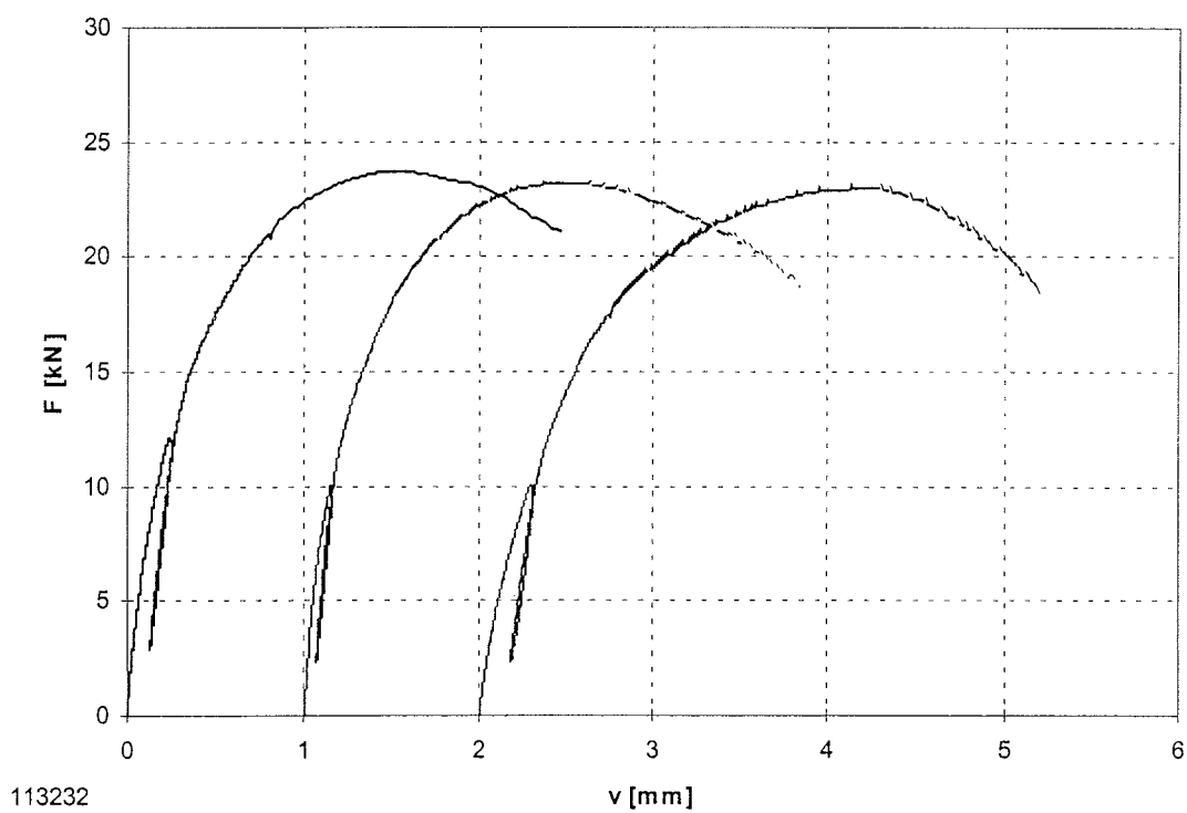
Bild B-81: Last-Verschiebungsdiagramm der Versuchsreihe 113232
