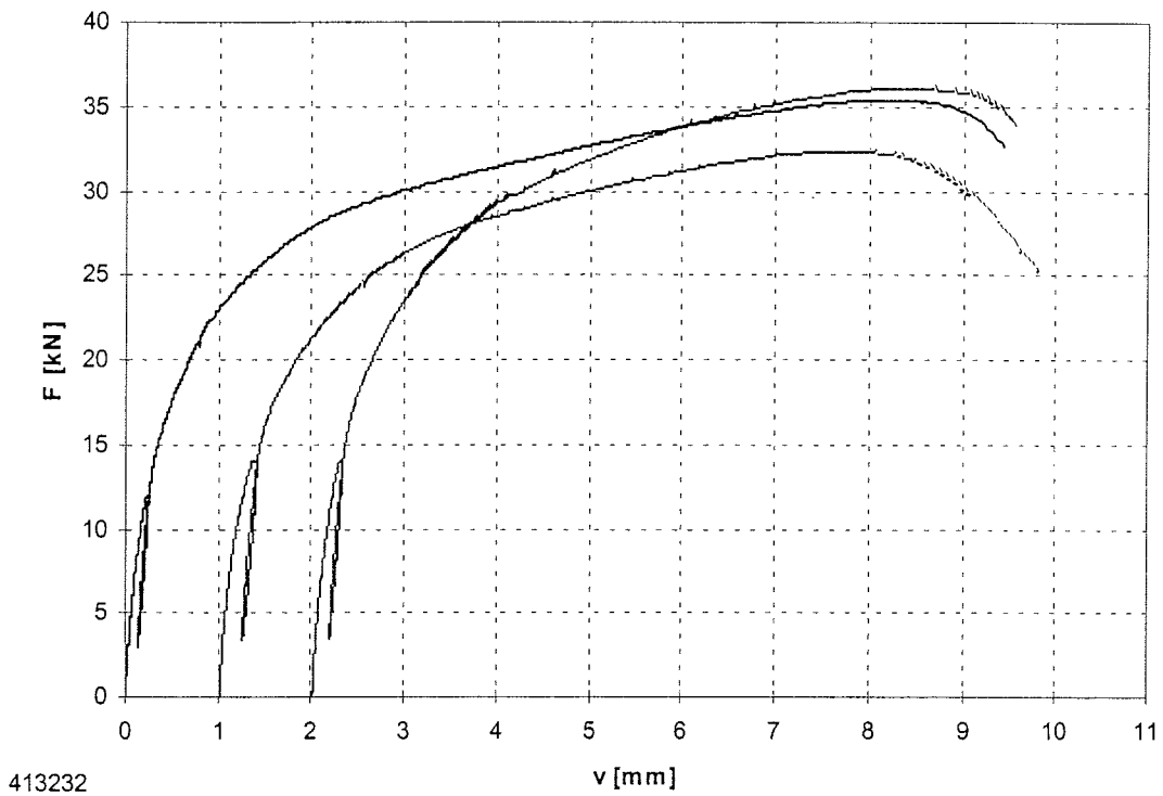
Bild B-93: Last-Verschiebungsdiagramm der Versuchsreihe 413232
