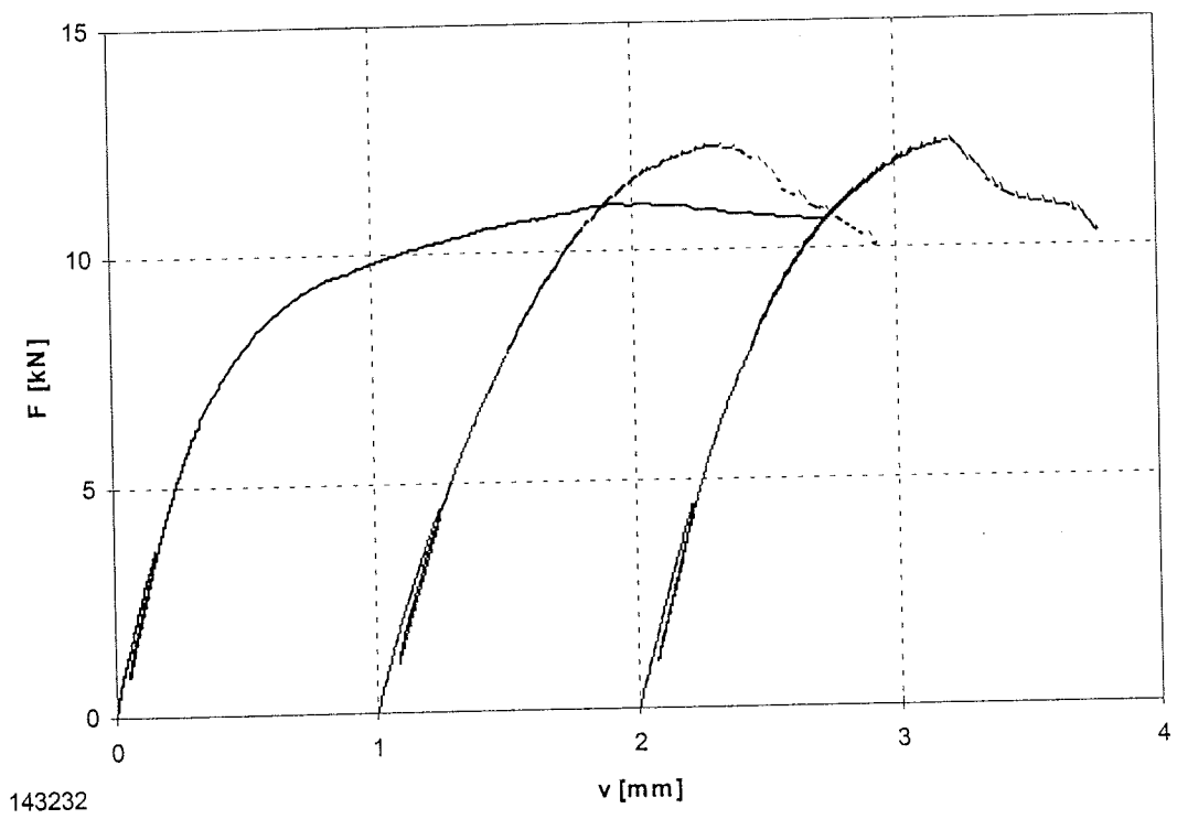
Bild B-84: Last-Verschiebungsdiagramm der Versuchsreihe 143232
