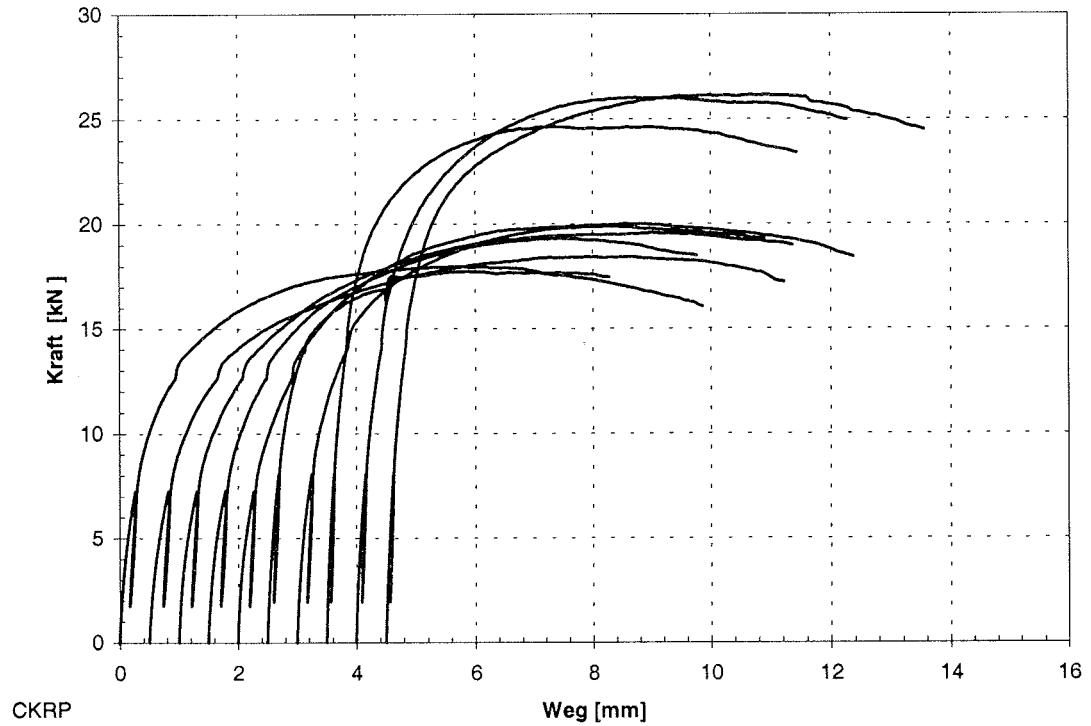
Abb. C-42: Last-Verschiebungs-Diagramm der Reihe CKRP
