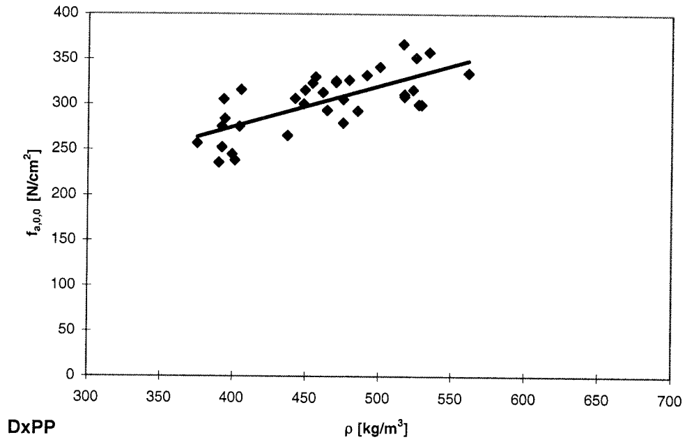
Abb. D-13: Nageltragfähigkeit-Rohdichte-Abhängigkeit der Reihen D-7
