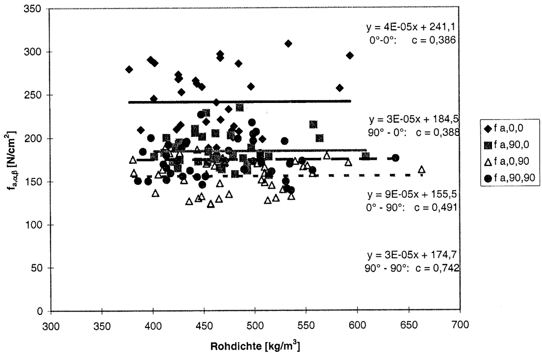
Abb. D-20: Umgerechnete Nageltragfähigkeitswerte in Abhängigkeit von der Rohdichte für Nagelplatte A
