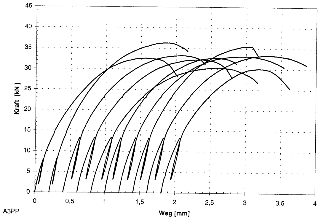
Abb. C-1: Last-Verschiebungs-Diagramm der Reihe A3PP
