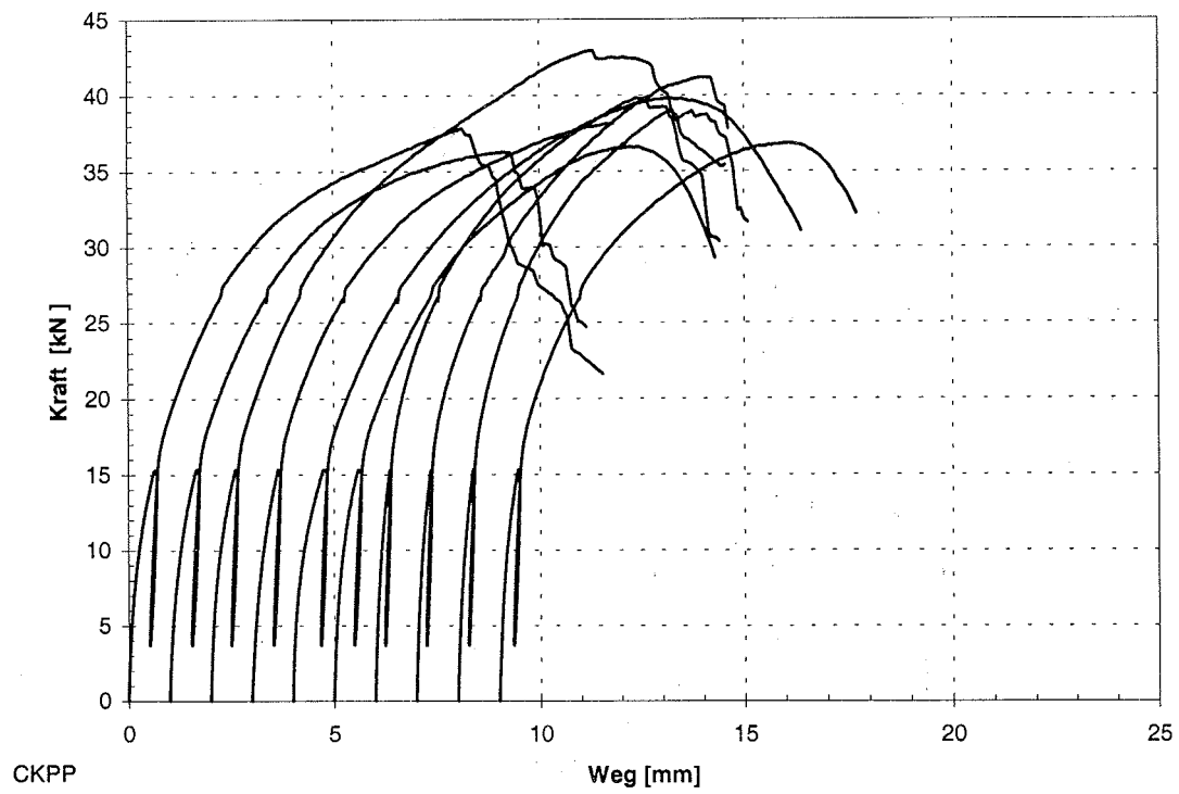
Abb. C-38: Last-Verschiebungs-Diagramm der Reihe CKPP
