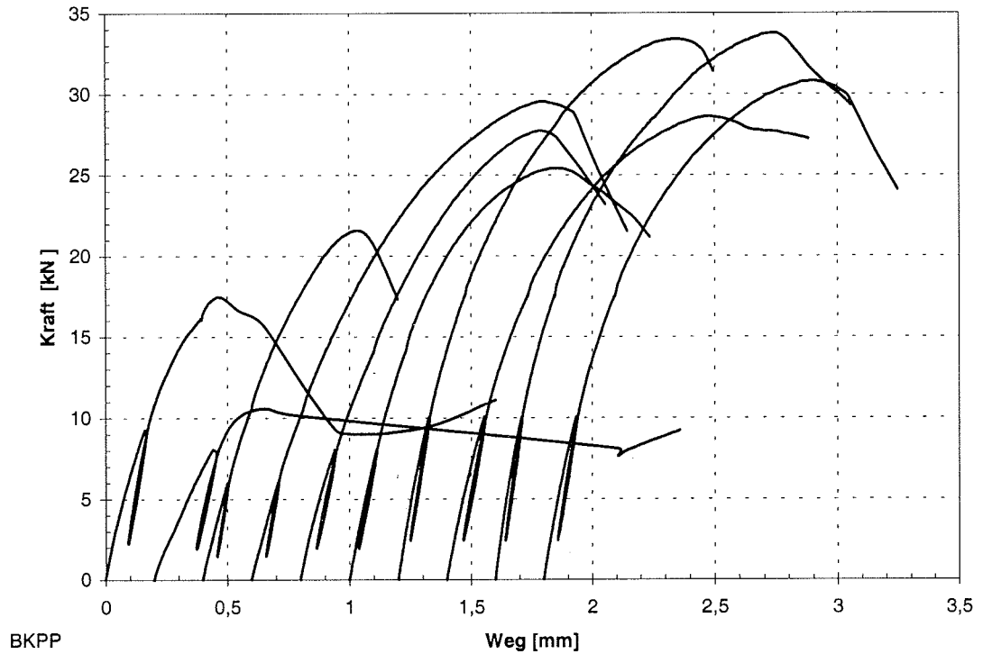
Abb. C-22: Last-Verschiebungs-Diagramm der Reihe BKPP
