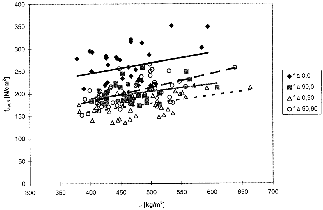
Abb. D-19: Vergleich der Abhängigkeiten für Nagelplatte A
