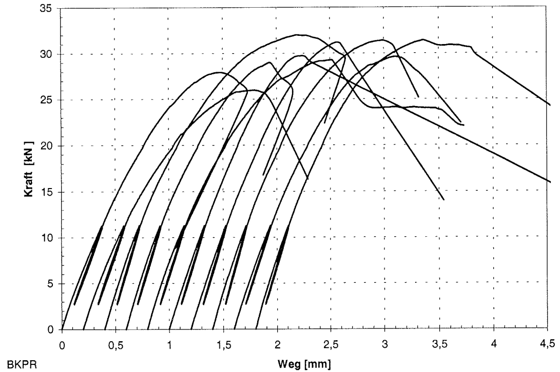
Abb. C-30: Last-Verschiebungs-Diagramm der Reihe BKPR
