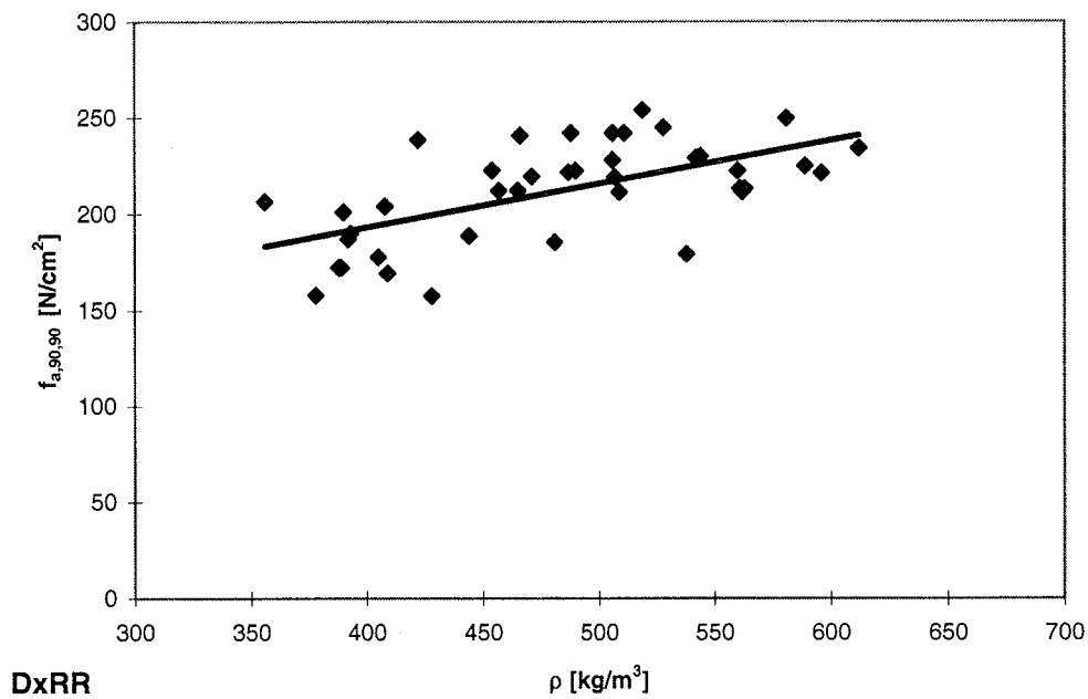
Abb. D-16: Nageltragfähigkeit-Rohdichte-Abhängigkeit der Reihen D-RR
