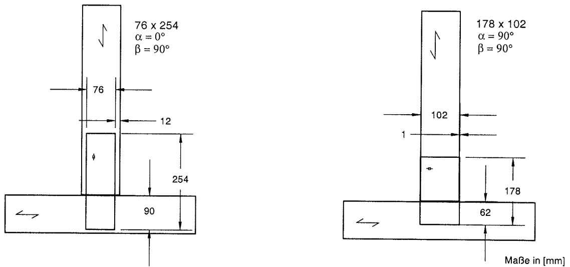
Abb. A-7: Form und Abmessungen der Versuchskörper der Reihe B
