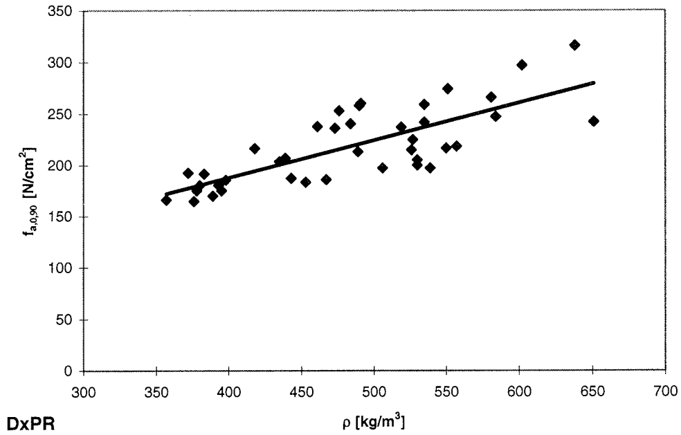
Abb. D-15: Nageltragfähigkeit-Rohdichte-Abhängigkeit der Reihen D-PR
