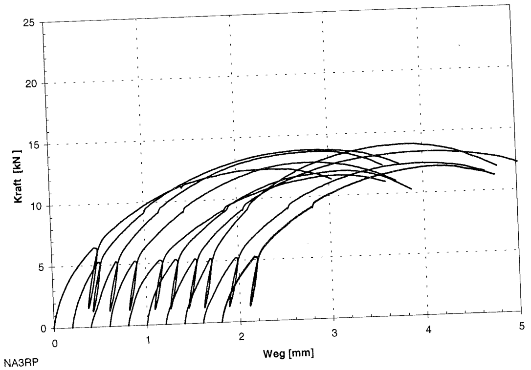
Abb. C-7: Last-Verschiebungs-Diagramm der Reihe NA3RP
