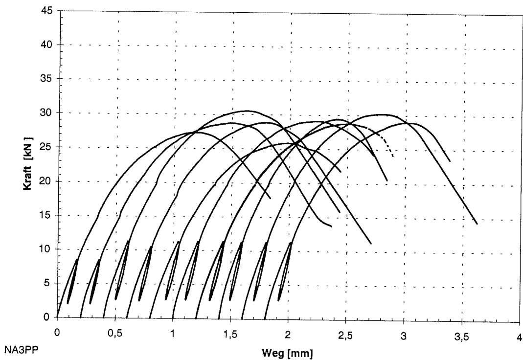
Abb. C-2: Last-Verschiebungs-Diagramm der Reihe NA3PP
