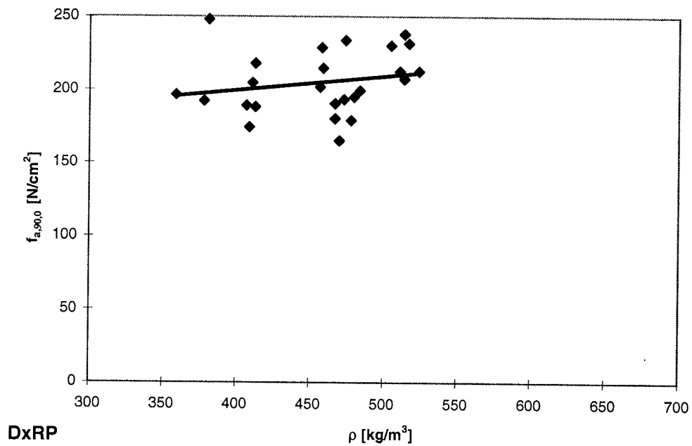
Abb. D-14: Nageltragfähigkeit-Rohdichte-Abhängigkeit der Reihen D-14
