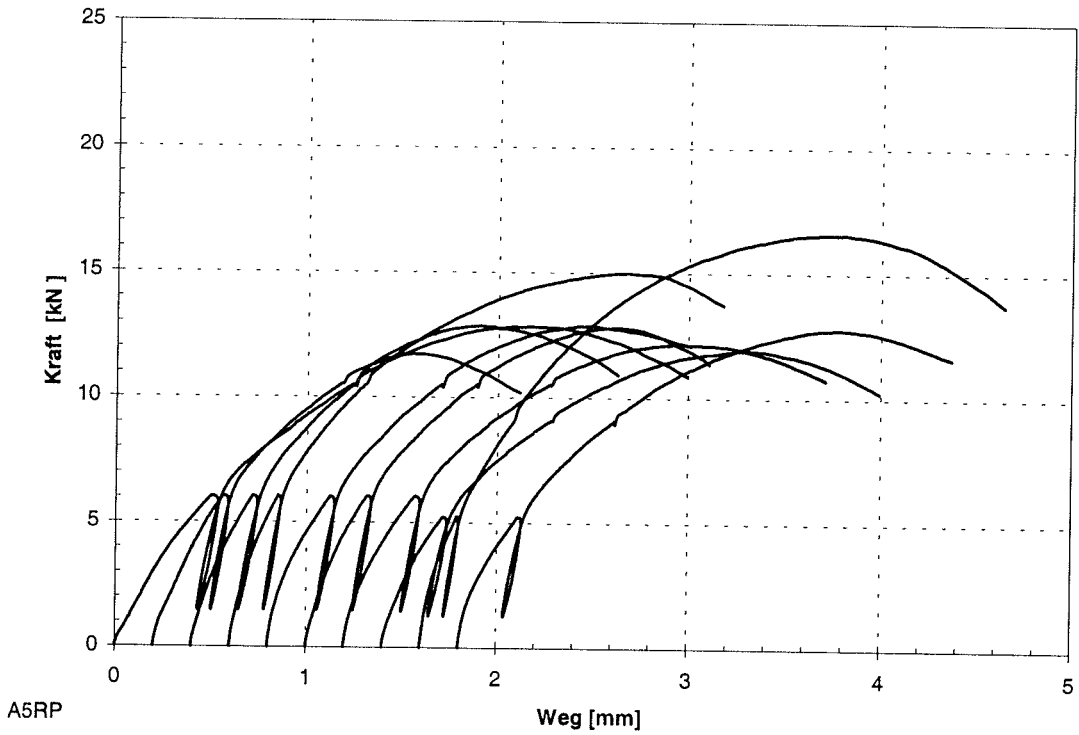
Abb. C-9: Last-Verschiebungs-Diagramm der Reihe A5RP
