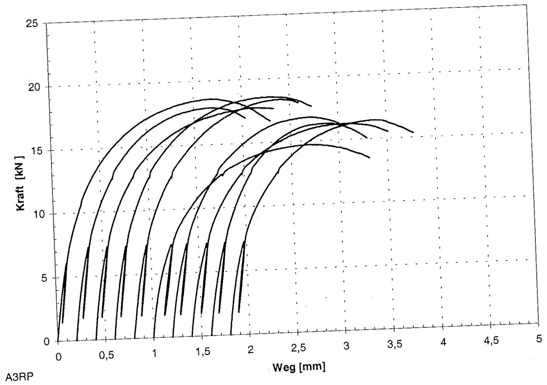
Abb. C-6: Last-Verschiebungs-Diagramm der Reihe A3RP
