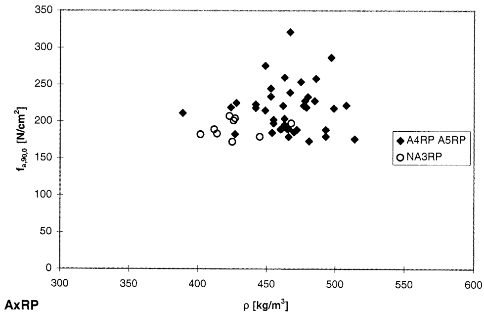
Abb. 4-5: Versuchsergebnisse Reihen NA3RP, A4RP und A5RP
