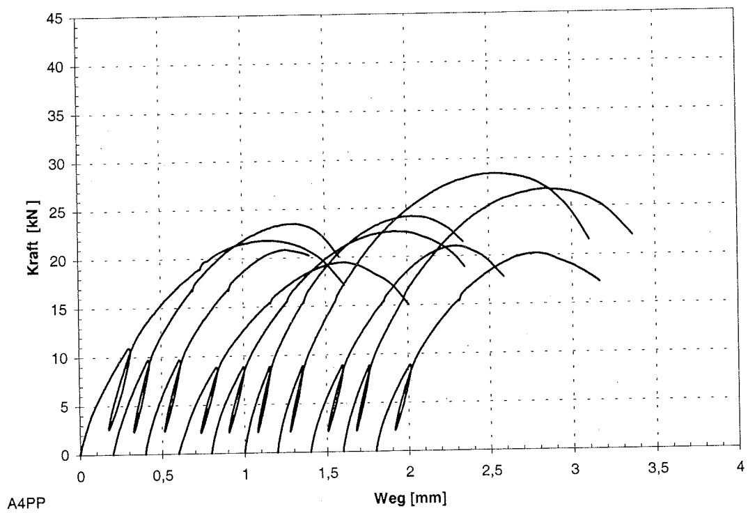
Abb. C-3: Last-Verschiebungs-Diagramm der Reihe A4PP
