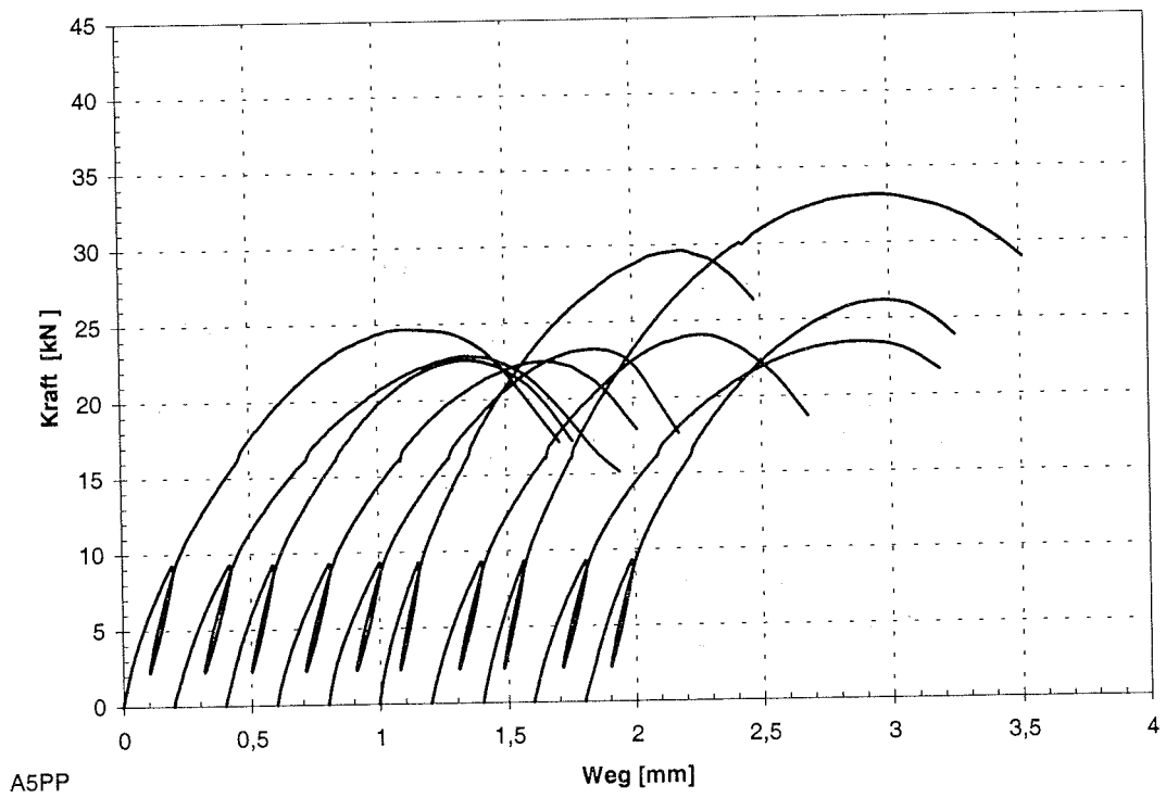
Abb. C-4: Last-Verschiebungs-Diagramm der Reihe A5PP
