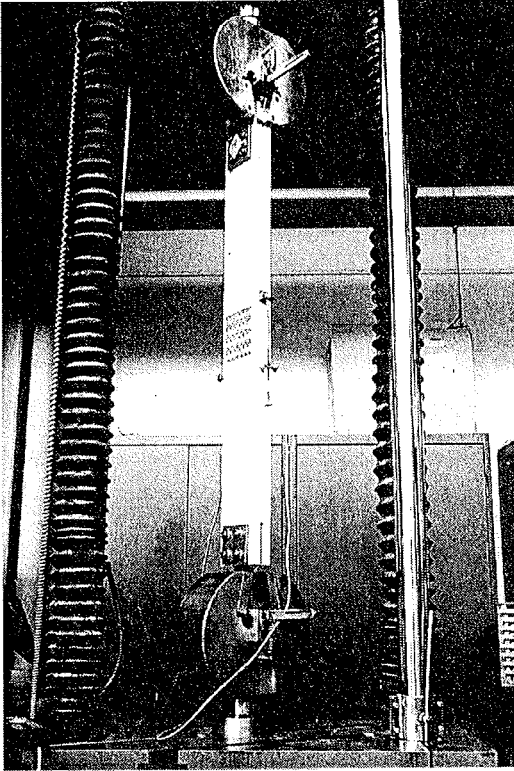
Abb. 3-2: Versuchsaufbau für Prüfkörper mit Belastung parallel (links) und rechtwinklig (rechts) zur Faserrichtung
