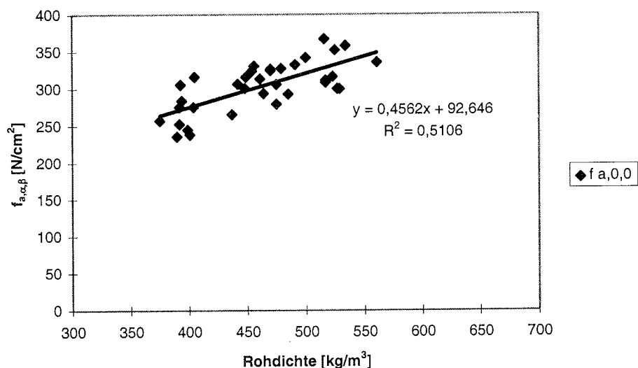
Abb. 4-7: Lineare Regression für Reihe DxPP
