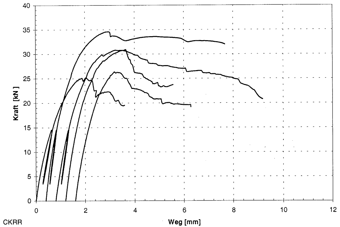
Abb. C-50: Last-Verschiebungs-Diagramm der Reihe CKRR
