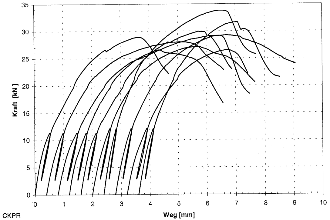
Abb. C-46: Last-Verschiebungs-Diagramm der Reihe CKPR
