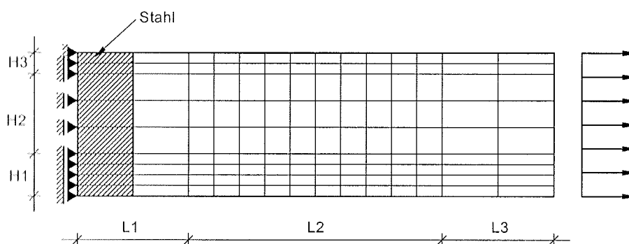
Bild 2: Unterteilung, Lastanordnung und Auflagerung eines Zugprüfkörpers
