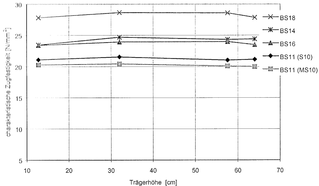
Bild 5: Einfluß der Trägerhöhe
