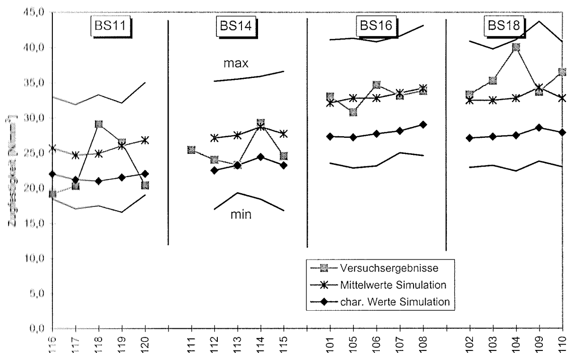
Bild 4: Vergleich Simulationen und Versuchsergebnisse der Hauptversuche
