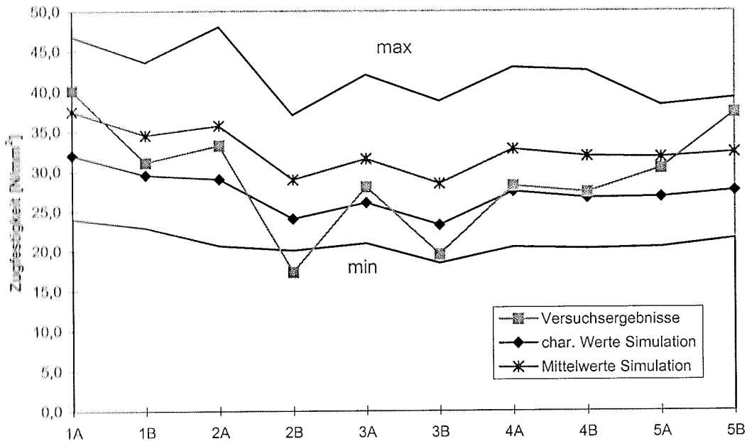
Bild 3: Vergleich Simulationen und Versuchsergebnisse der Vorversuche
