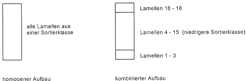
Bild 8: Homogen und kombiniert aufgebauter Träger
