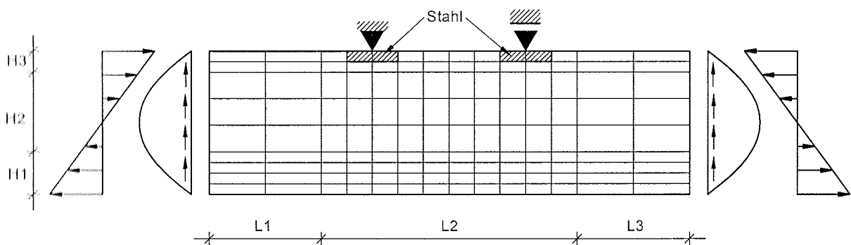
Bild 1: Unterteilung, Lastanordnung und Auflagerung eines Biegeträgers nach COLLING (1992)
