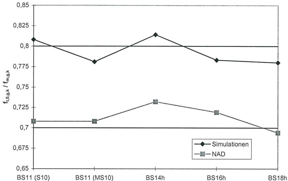
Bild 9: Verhältnis Zugfestigkeit zur Biegefestigkeit
