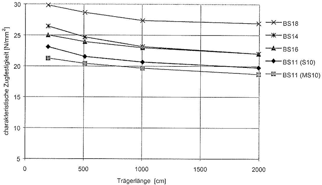
Bild 6: Einfluß der Trägerlänge
