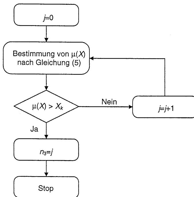
Abb. 2: Algorithmus zur Bestimmung des „Cutting Levels“ n_3
