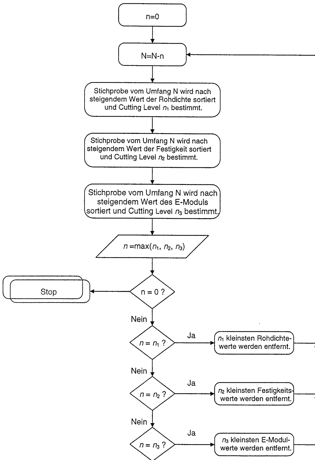
Abb. 1: Algorithmus für die Durchführung von „Optimal Ranking“
